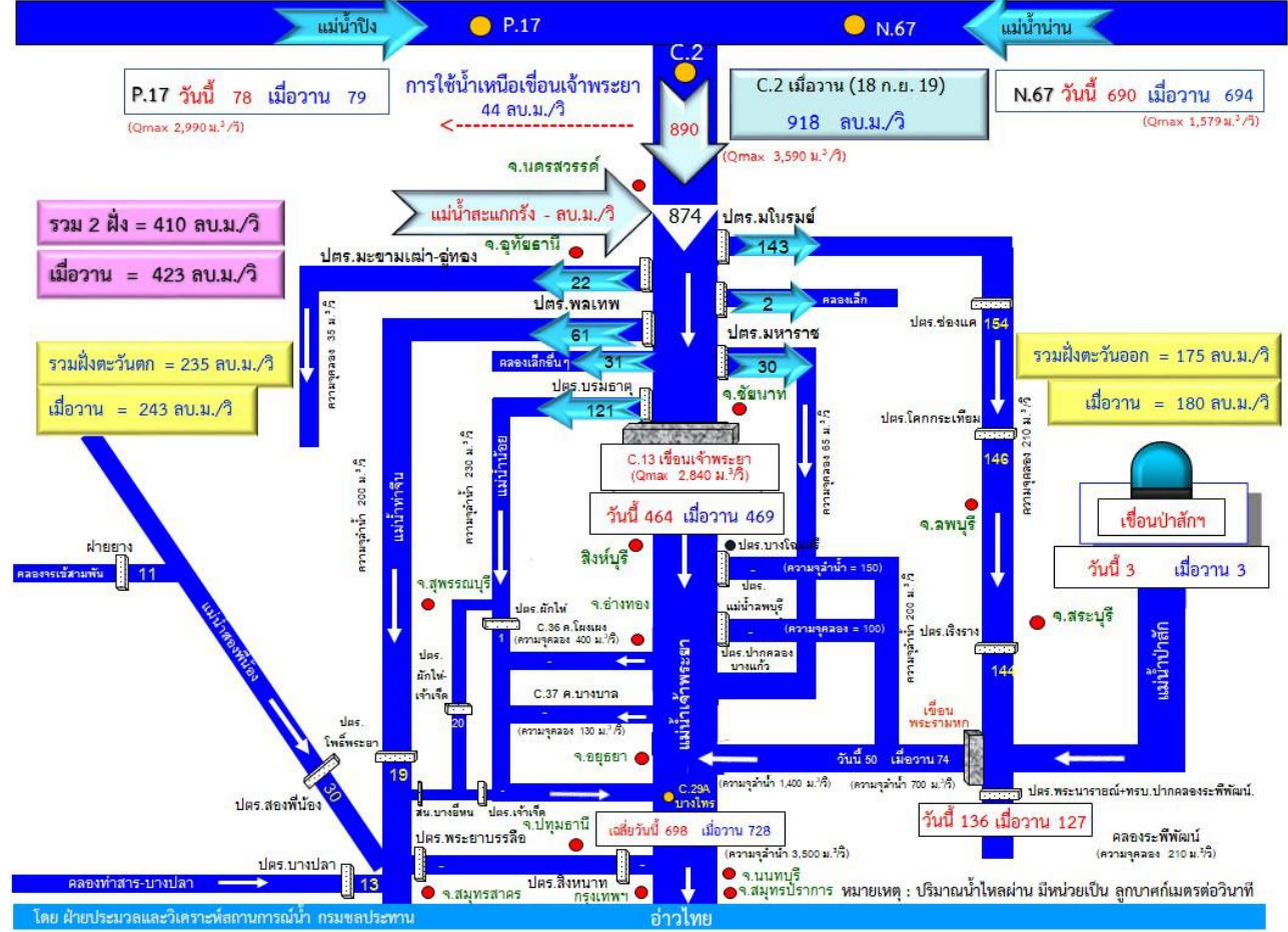
ข้อมูลสถานการณ์น้ำในแม่น้ำเจ้าพระยา (เวลา 06.00 น.) วันพฤหัสบดี 19 กันยายน 2562
