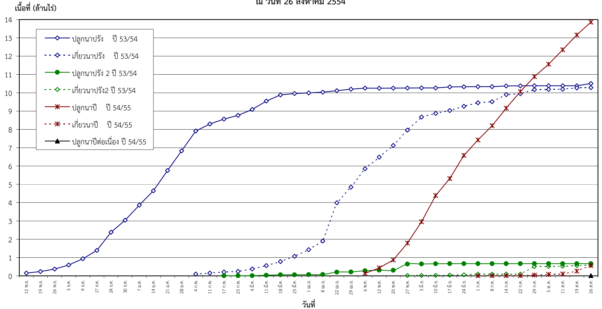
กราฟแสดง เนื้อที่ปลูก และเนื้อที่เก็บเกี่ยวข้าว ในเขตชลประทาน ปีเพาะปลูก 2553/54 - 2554/55 ณ วันที่ 26 สิงหาคม 2554
