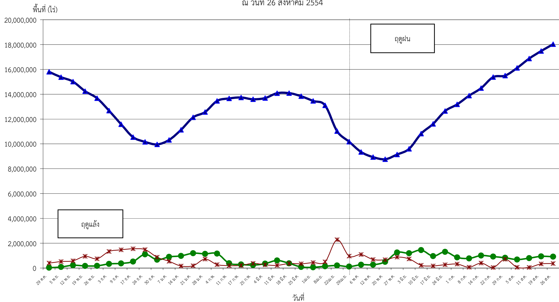
กราฟแสดงสภาพการปลูกพืชทุกชนิด ในเขตโครงการชลประทานขนาดใหญ่และกลาง เป็นรายสัปดาห์ ณ วันที่ 26 สิงหาคม 2554
