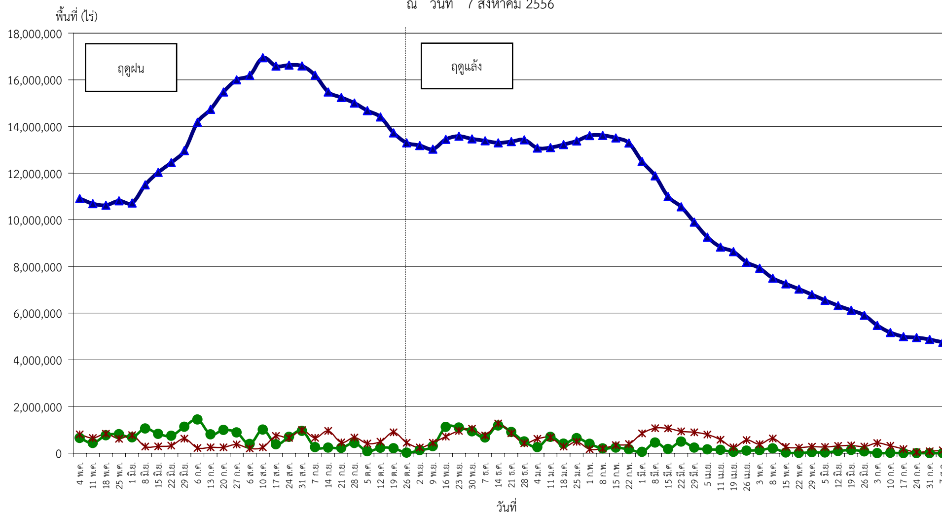
กราฟแสดงสภาพการปลูกพืชทุกชนิด ในเขตโครงการชลประทานขนาดใหญ่และกลาง เป็นรายสัปดาห์ ณ วันที่ 7 สิงหาคม 2556
