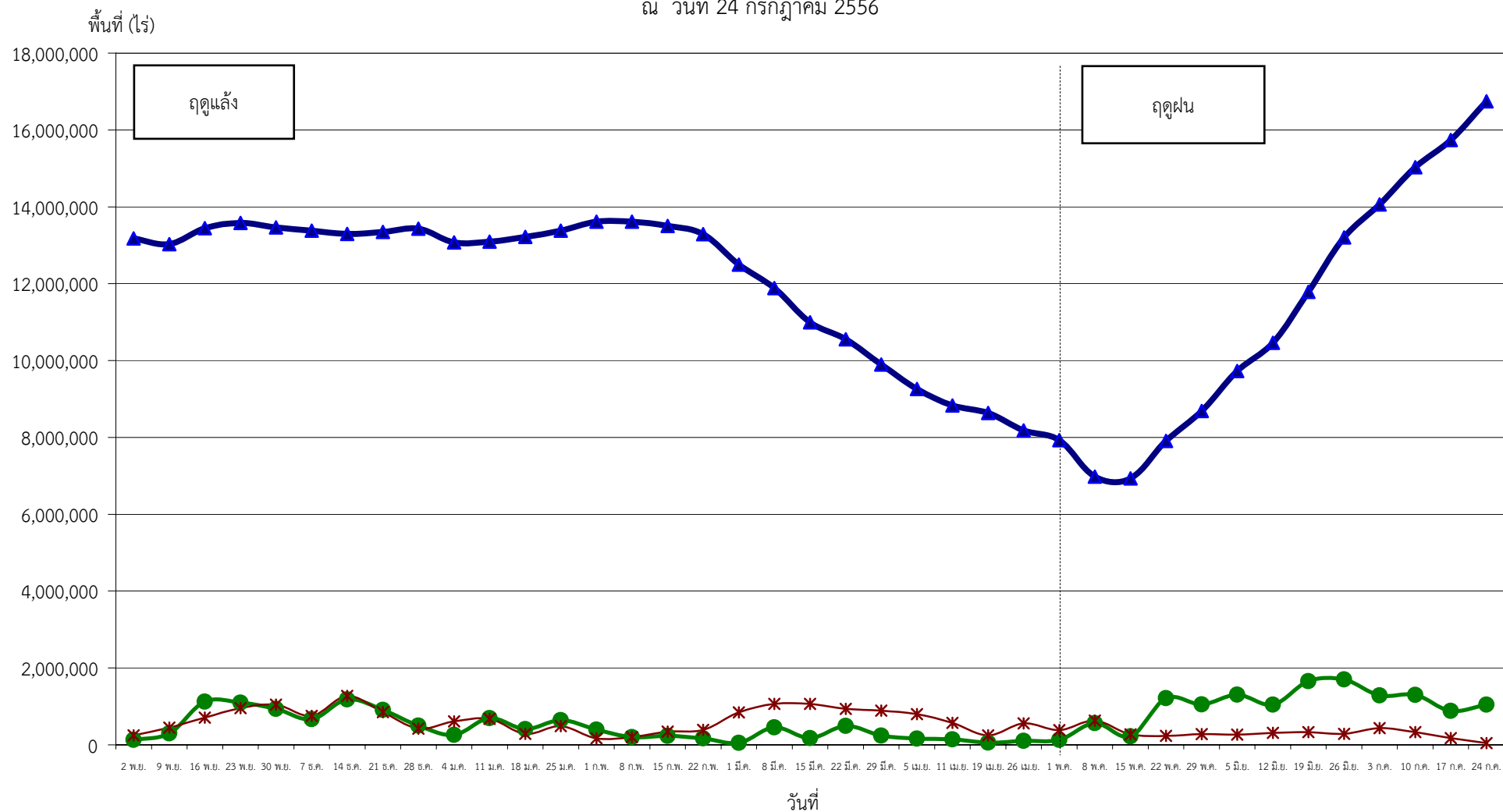
กราฟแสดงสภาพการปลูกพืชทุกชนิด ในเขตโครงการชลประทานขนาดใหญ่และกลาง เป็นรายสัปดาห์ ณ วันที่ 24 กรกฎาคม 2556
