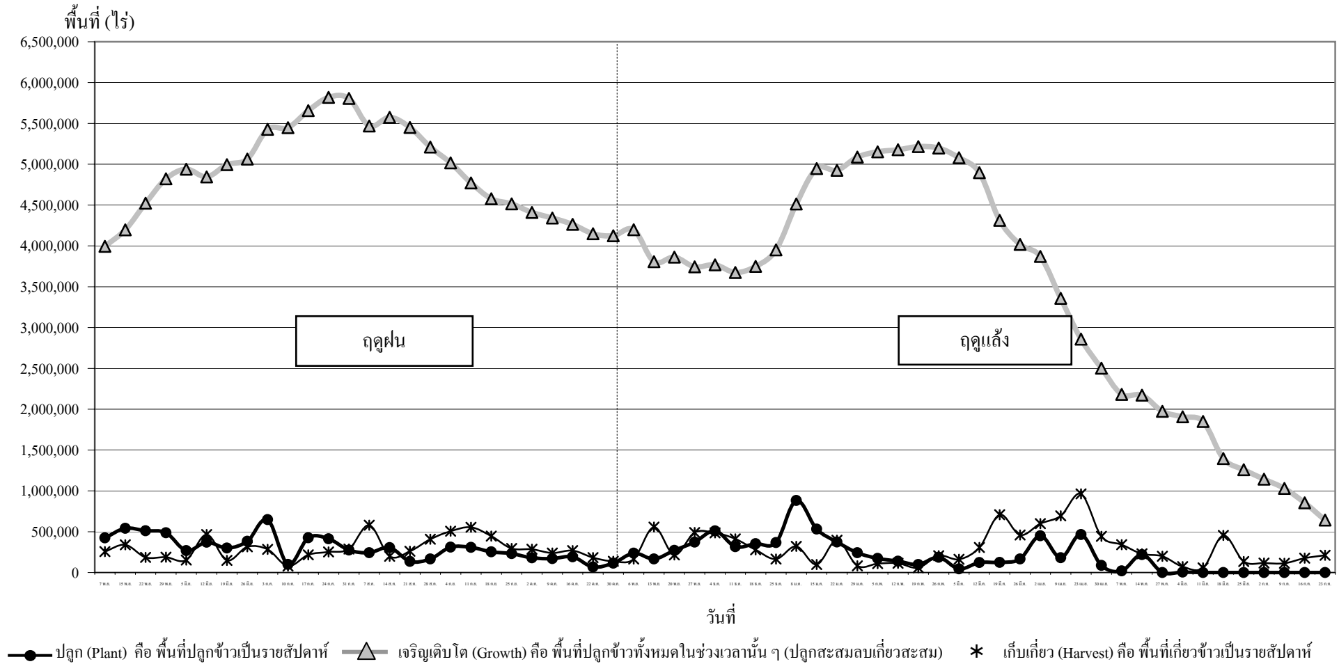
กราฟแสดงสภาพการปลูกข้าว ในเขตลุ่มน้ำเจ้าพระยาทำอย่างเก็บน้ำเขื่อนภูมิพลและสิริกิติ์ เป็นรายสัปดาห์ ณ วันที่ 23 กรกฎาคม 2553
