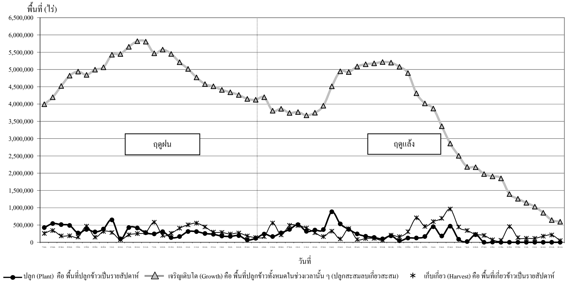
กราฟแสดงสภาพการปลูกข้าว ในเขตลุ่มน้ำเจ้าพระยาทำอย่างเก็บน้ำเขื่อนภูมิพลและสิริกิติ์ เป็นรายสัปดาห์ ณ วันที่ 30 กรกฎาคม 2553
