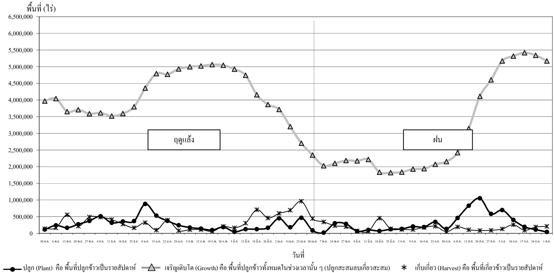
กราฟแสดงสภาพการปลูกข้าว ในเขตลุ่มน้ำเจ้าพระยาทำอย่างเก็บน้ำเขื่อนภูมิพลและสิริกิติ์ เป็นรายสัปดาห์ ณ วันที่ 1 ตุลาคม 2553
