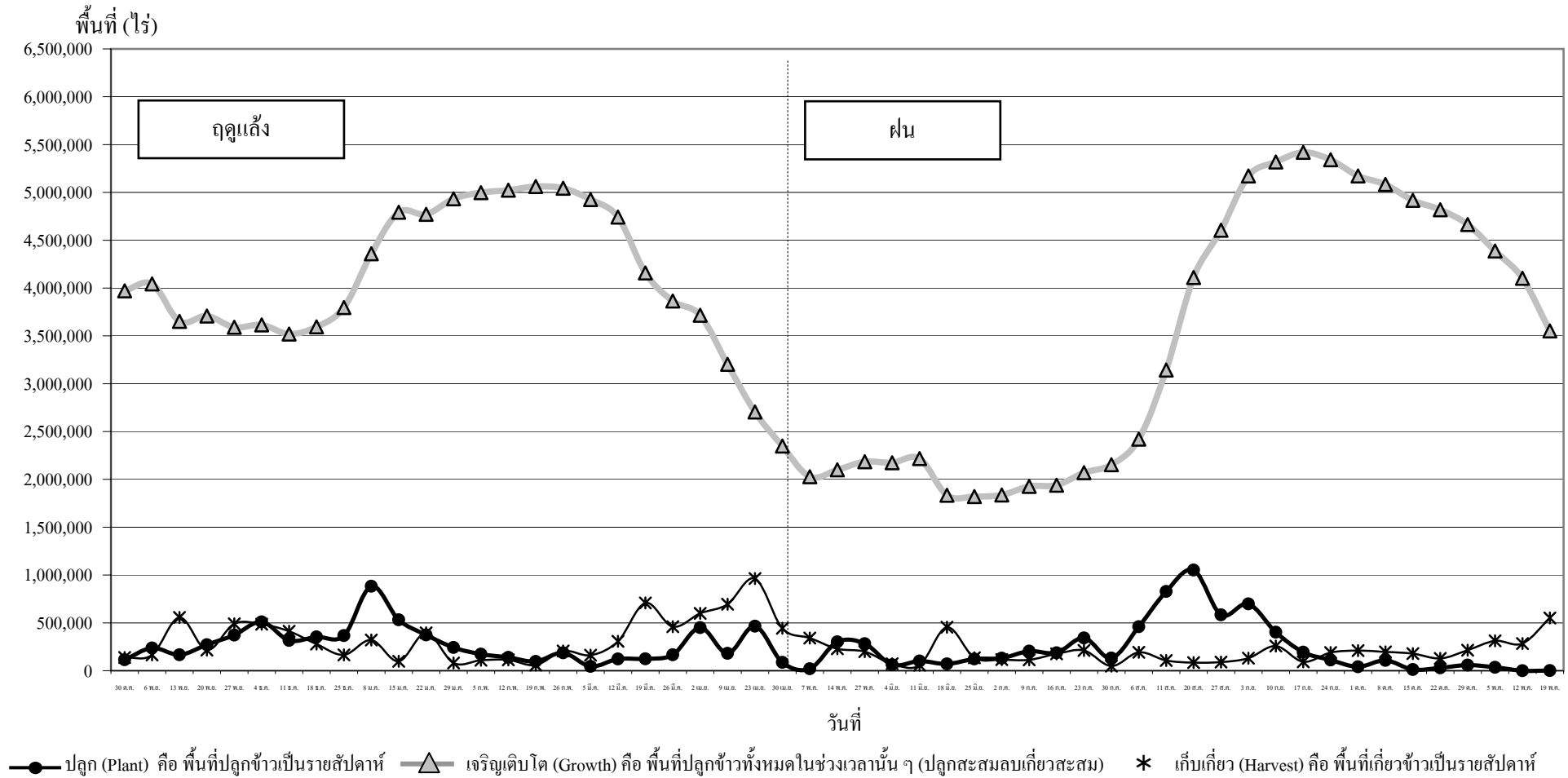
กราฟแสดงสภาพการปลูกข้าว ในเขตลุ่มน้ำเจ้าพระยาทำอย่างเก็บน้ำเขื่อนภูมิพลและสิริกิติ์ เป็นรายสัปดาห์ ณ วันที่ 19 พฤศจิกายน 2553
