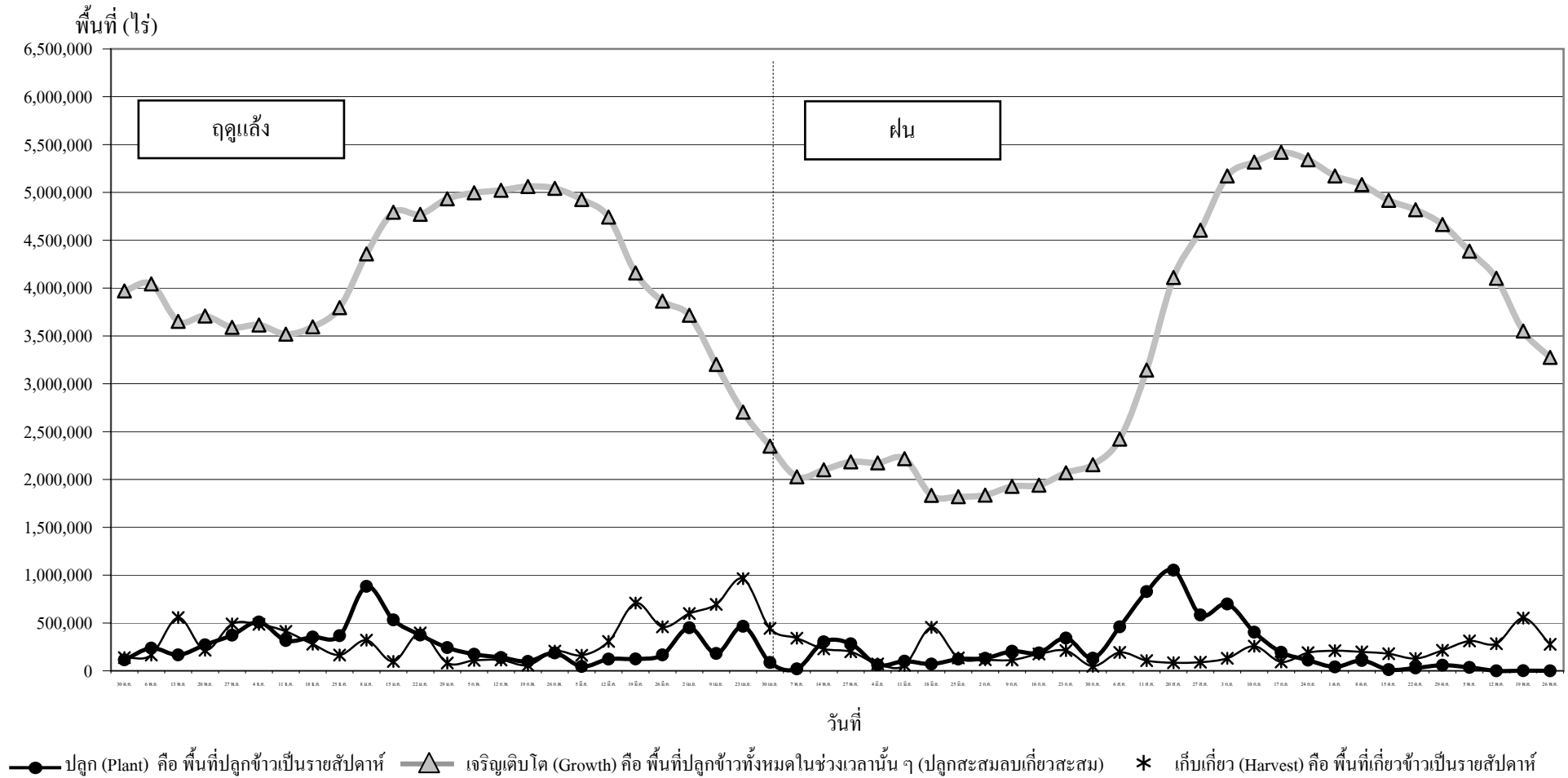
กราฟแสดงสภาพการปลูกข้าว ในเขตลุ่มน้ำเจ้าพระยาทำอย่างเก็บน้ำเขื่อนภูมิพลและสิริกิติ์ เป็นรายสัปดาห์ ณ วันที่ 26 พฤศจิกายน 2553
