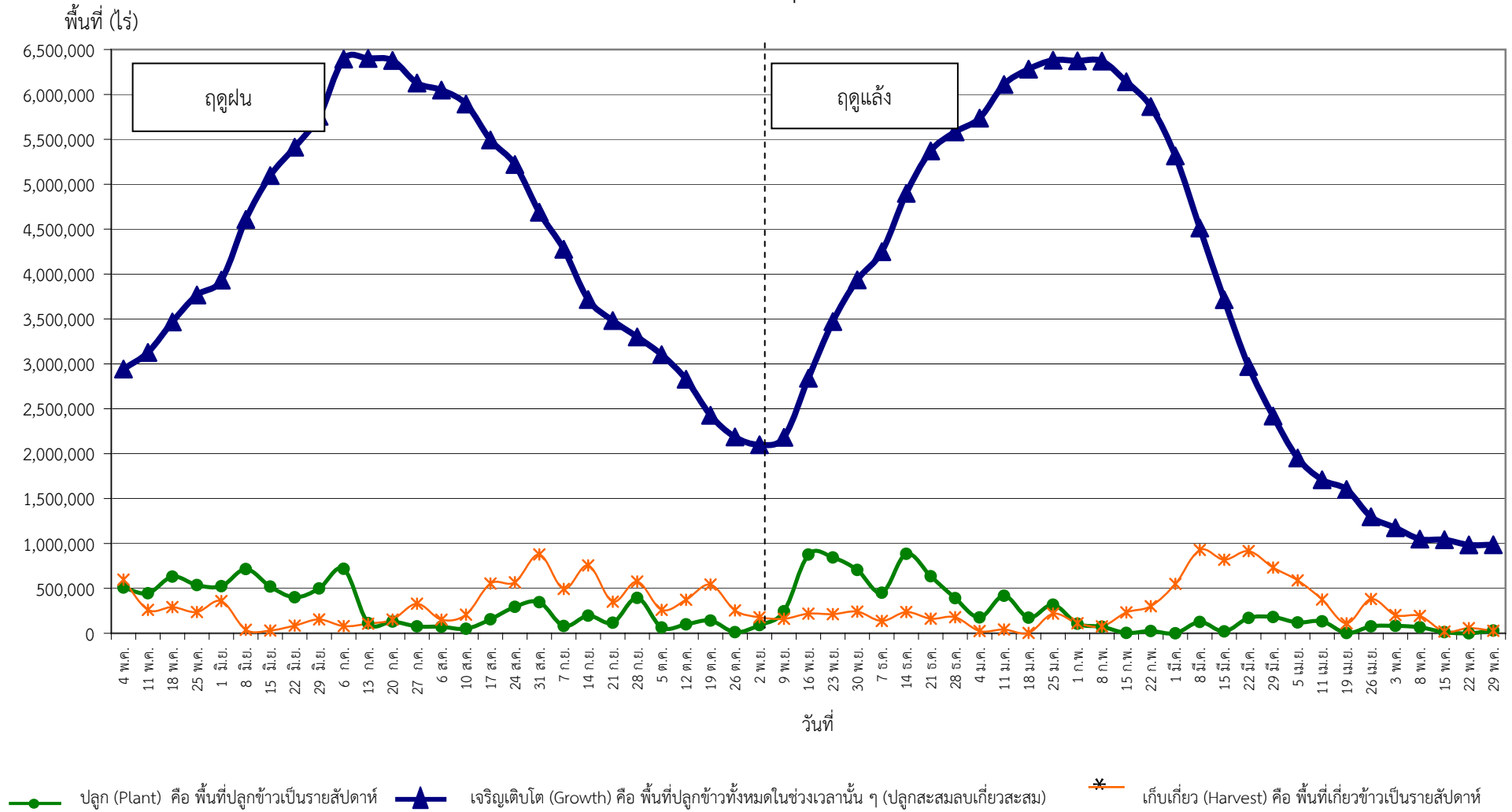
กราฟแสดงสภาพการปลูกข้าว ในเขตลุ่มน้ำเจ้าพระยาทำอย่างเก็บน้ำเขื่อนภูมิพลและสิริกิติ์ เป็นรายสัปดาห์ ณ วันที่ 29 พฤษภาคม 2556
