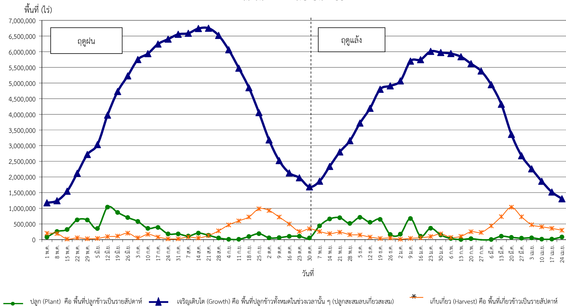
กราฟแสดงสภาพการปลูกข้าว ในเขตลุ่มน้ำเจ้าพระยาทำอย่างเก็บน้ำเขื่อนภูมิพลและสิริกิติ์ เป็นรายสัปดาห์ ณ วันที่ 24 เมษายน 2557
