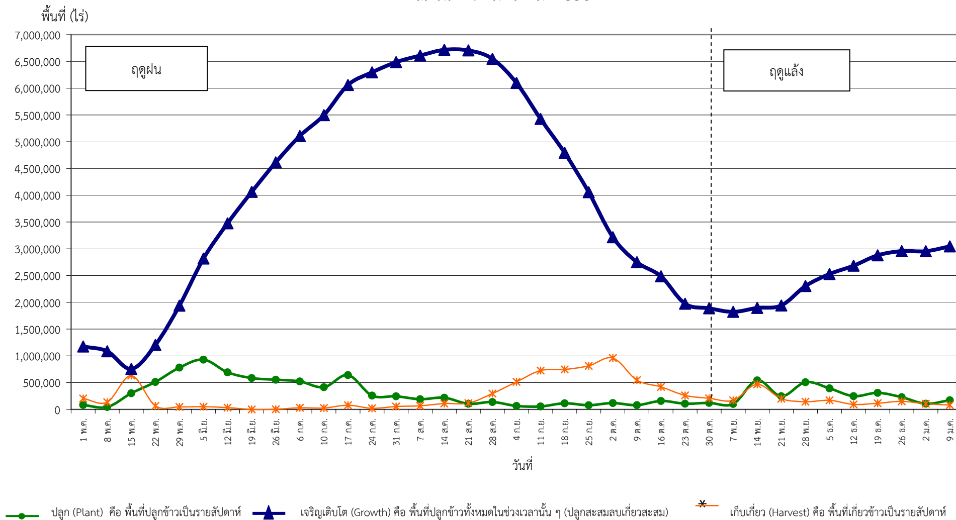
กราฟแสดงสภาพการปลูกข้าว ในเขตลุ่มน้ำเจ้าพระยาทำอย่างเก็บน้ำเขื่อนภูมิพลและสิริกิติ์ เป็นรายสัปดาห์ ณ วันที่ 9 มกราคม 2558
