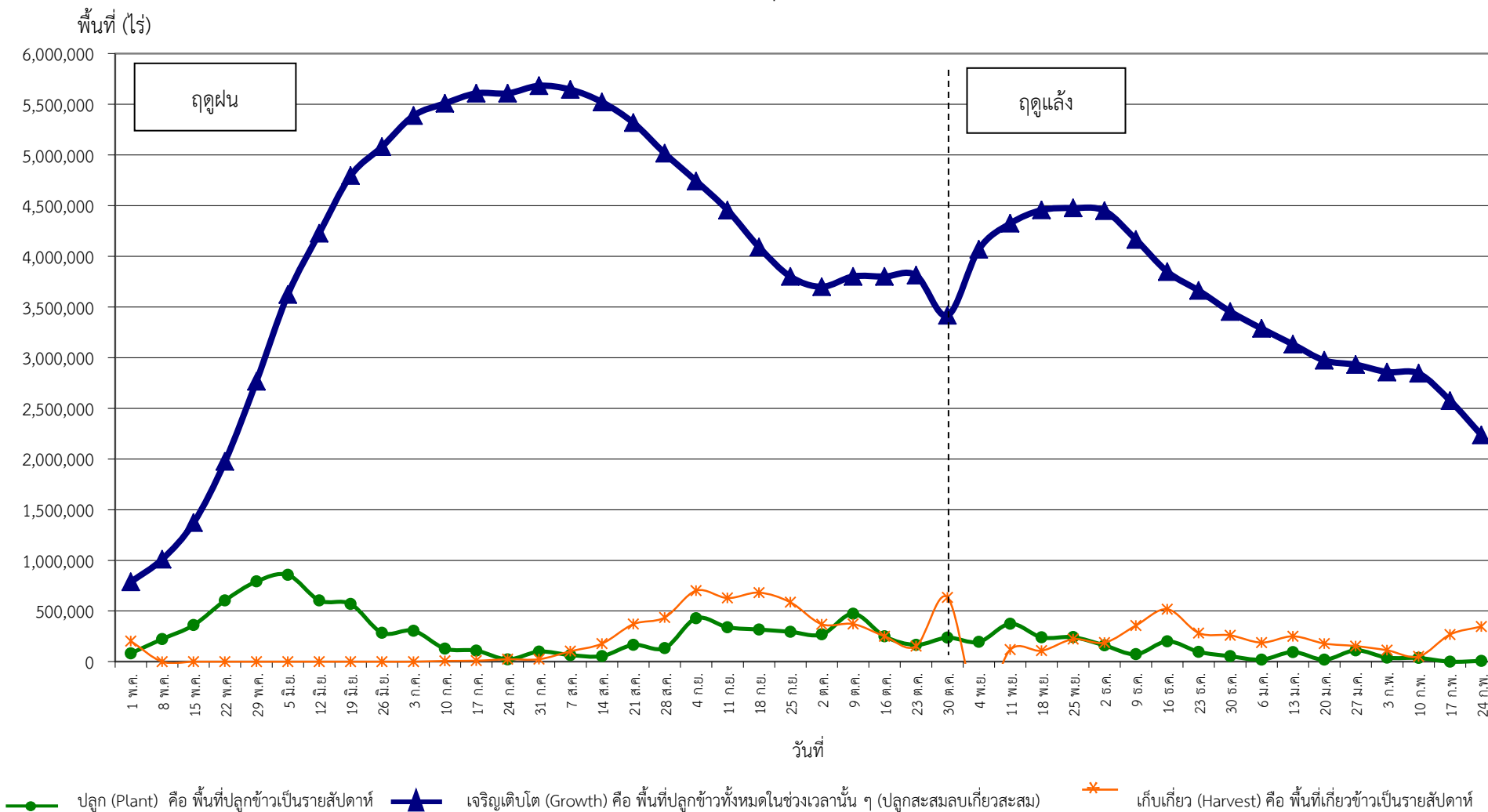
กราฟแสดงสภาพการปลูกข้าว ในเขตลุ่มน้ำเจ้าพระยาทำอย่างเก็บน้ำเขื่อนภูมิพลและสิริกิติ์ เป็นรายสัปดาห์ ณ วันที่ 24 กุมภาพันธ์ 2559
