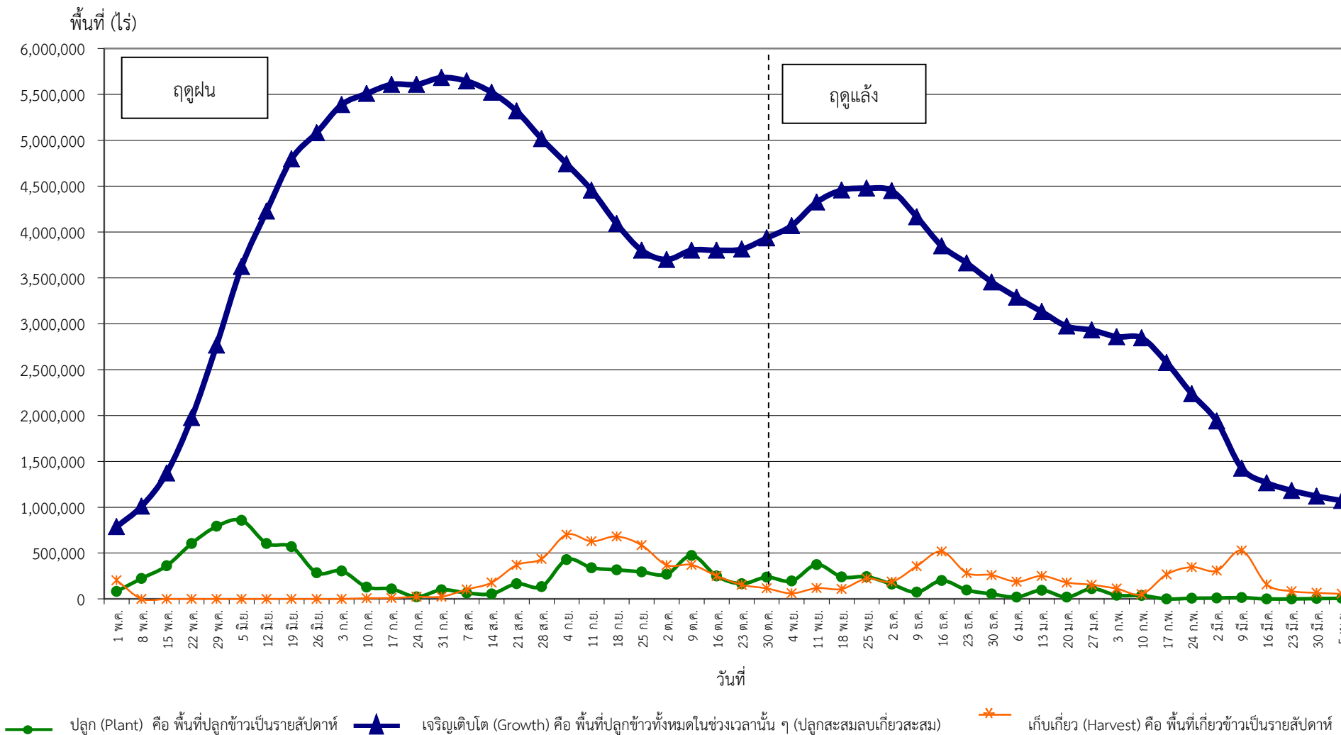
กราฟแสดงสภาพการปลูกข้าว ในเขตลุ่มน้ำเจ้าพระยาทำอย่างเก็บน้ำเขื่อนภูมิพลและสิริกิติ์ เป็นรายสัปดาห์ ณ วันที่ 5 เมษายน 2559
