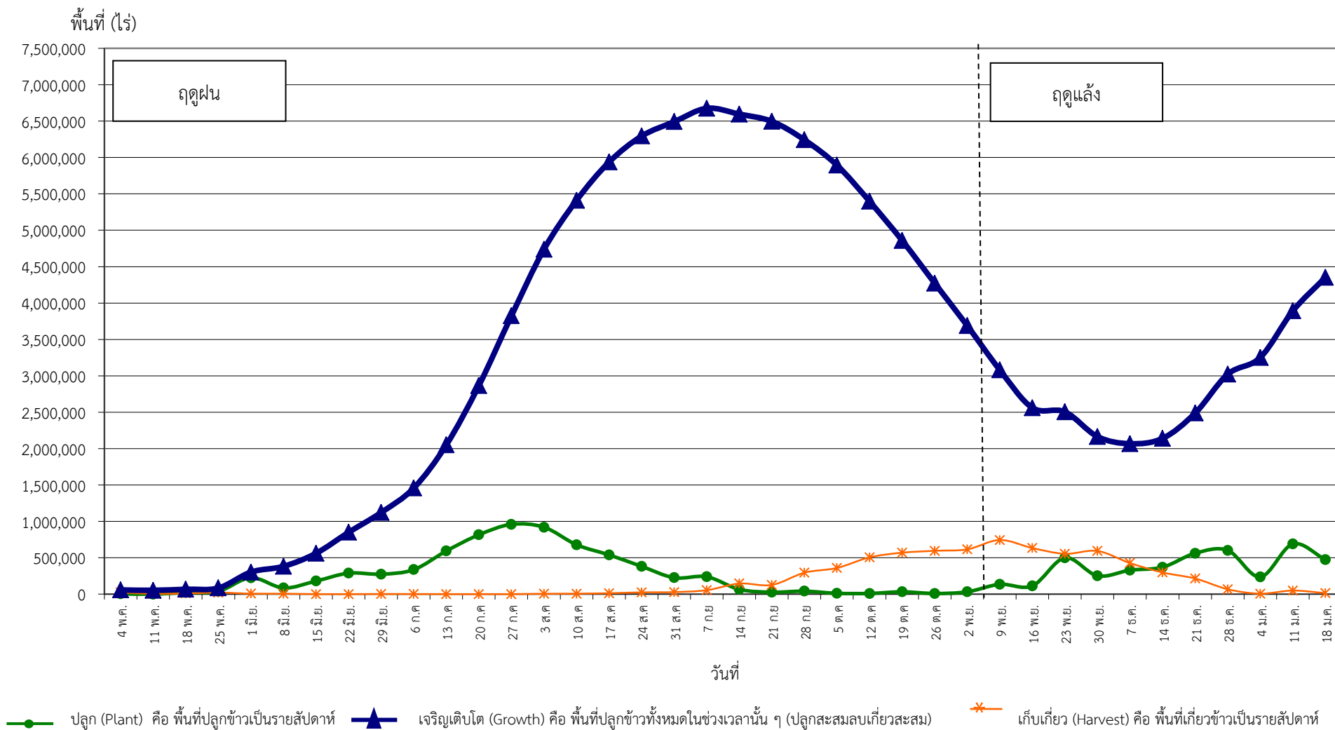
กราฟแสดงสภาพการปลูกข้าว ในเขตลุ่มน้ำเจ้าพระยาทำอย่างเก็บน้ำเขื่อนภูมิพลและสิริกิติ์ เป็นรายสัปดาห์ ณ วันที่ 18 มกราคม 2560
