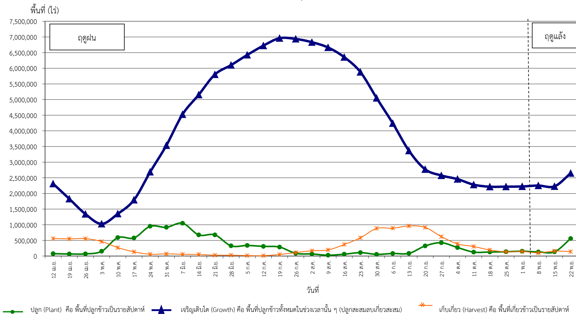
กราฟแสดงสภาพการปลูกข้าว ในเขตลุ่มน้ำเจ้าพระยาทำอย่างเก็บน้ำเขื่อนภูมิพลและสิริกิติ์ เป็นรายสัปดาห์ ณ วันที่ 22 พฤศจิกายน 2560
