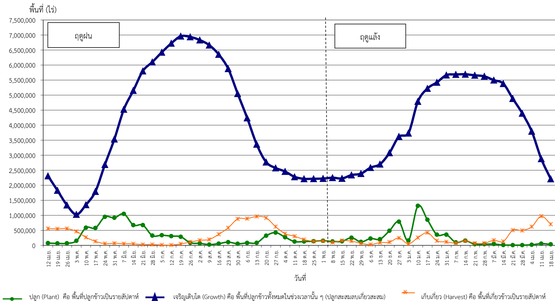
กราฟแสดงสภาพการปลูกข้าว ในเขตลุ่มน้ำเจ้าพระยาทำอย่างเก็บน้ำเขื่อนภูมิพลและสิริกิติ์ เป็นรายสัปดาห์ ณ วันที่ 18 เมษายน 2561
