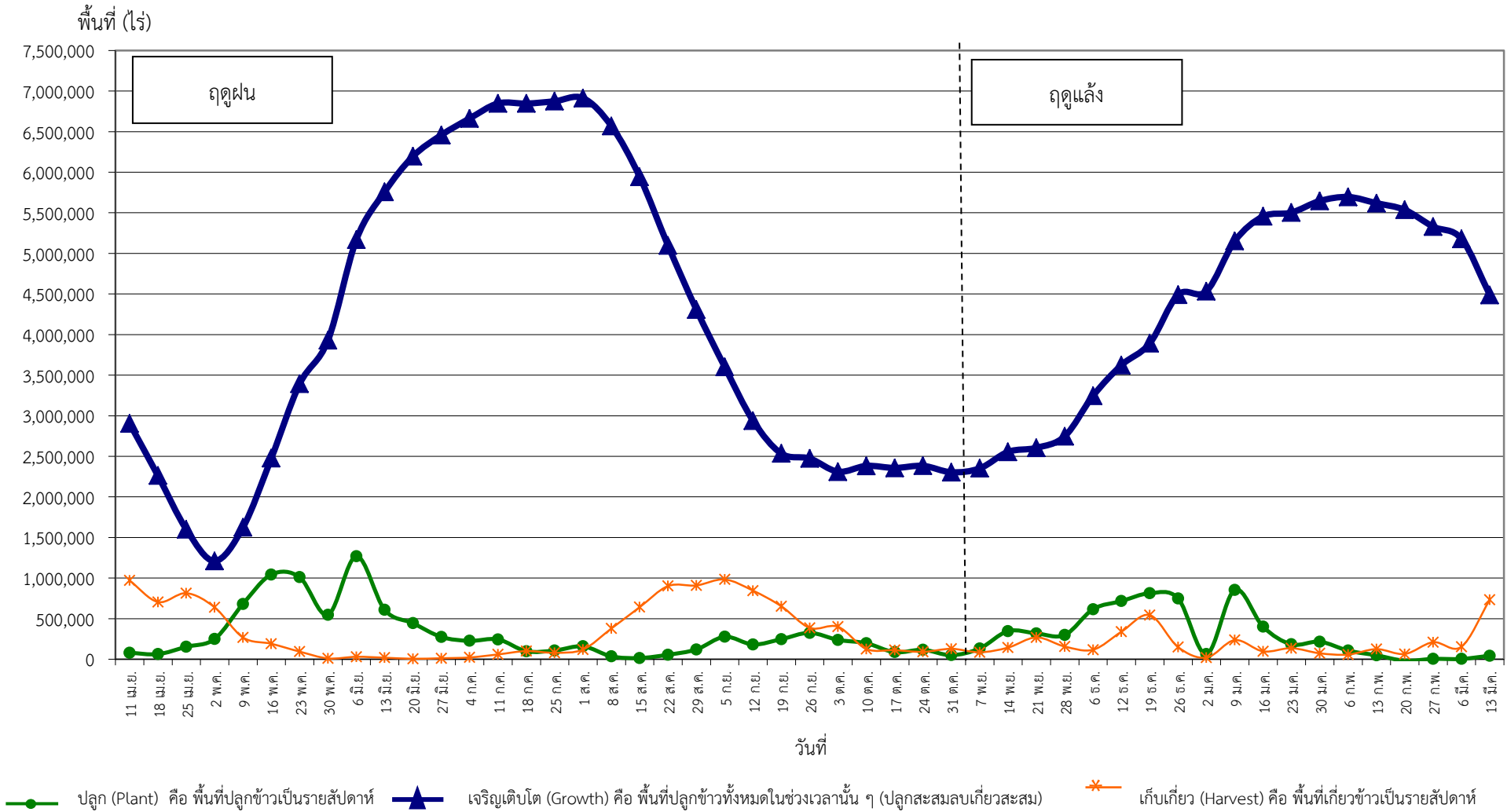
กราฟแสดงสภาพการปลูกข้าว ในเขตลุ่มน้ำเจ้าพระยาทำอย่างเก็บน้ำเขื่อนภูมิพลและสิริกิติ์ เป็นรายสัปดาห์ ณ วันที่ 13 มีนาคม 2562
