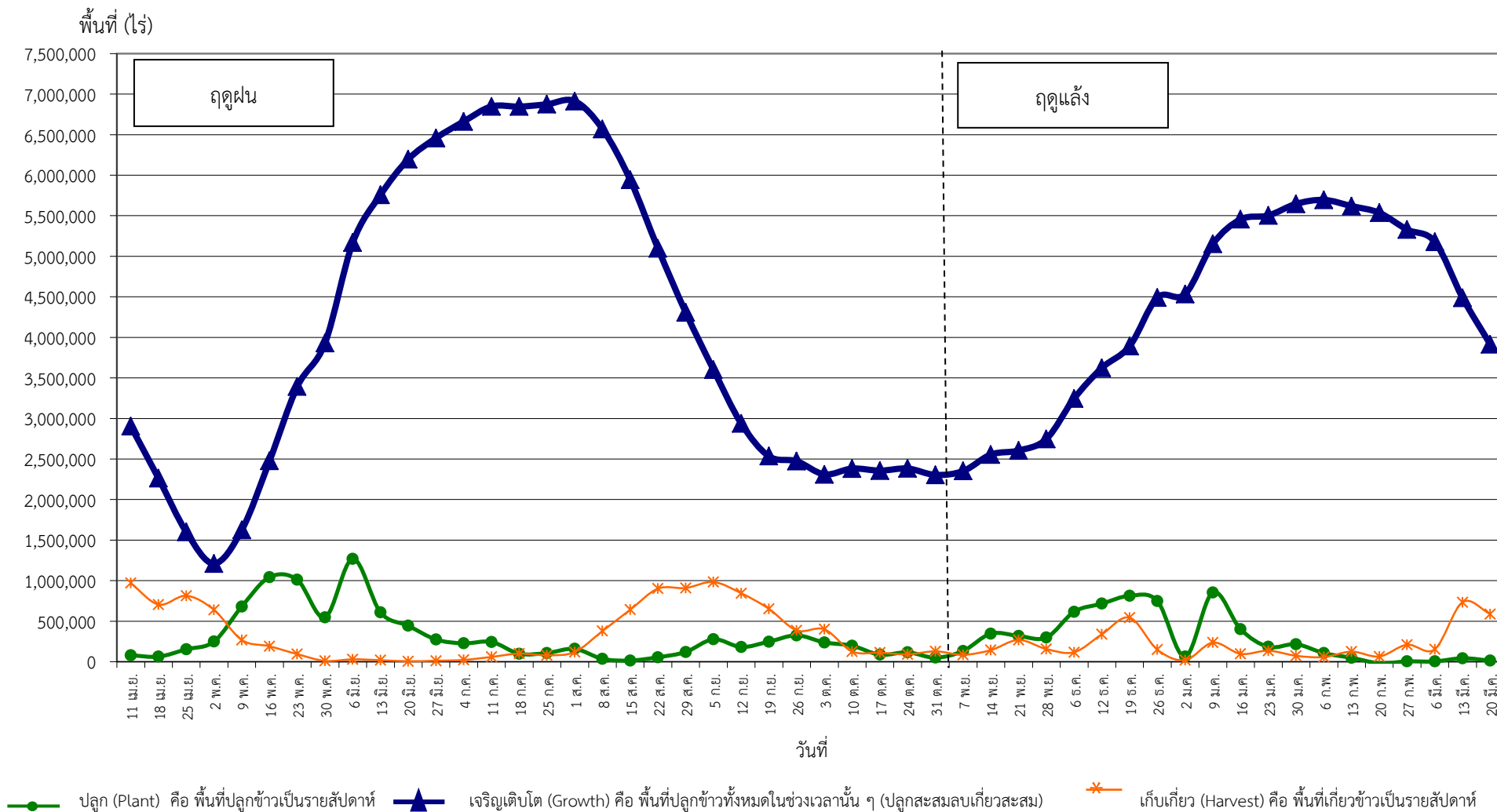
กราฟแสดงสภาพการปลูกข้าว ในเขตลุ่มน้ำเจ้าพระยาทำอย่างเก็บน้ำเขื่อนภูมิพลและสิริกิติ์ เป็นรายสัปดาห์ ณ วันที่ 20 มีนาคม 2562
