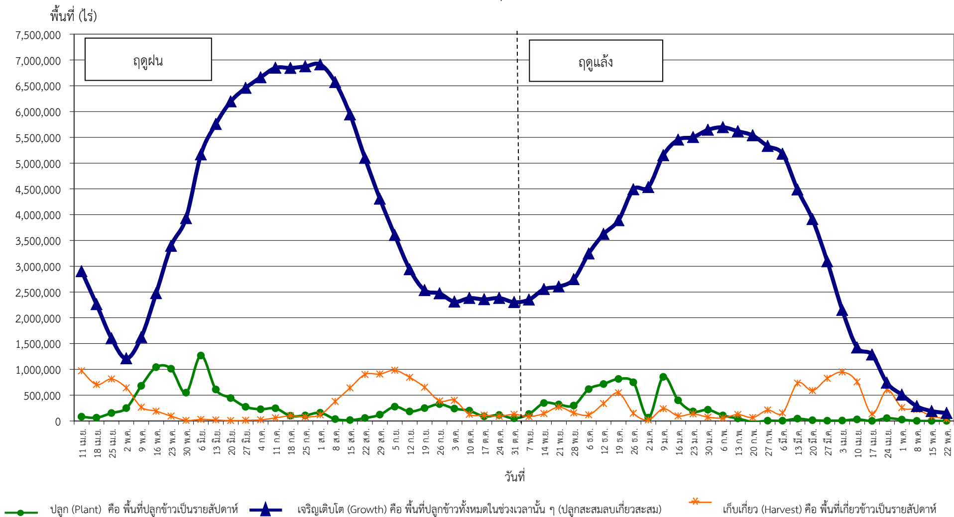
กราฟแสดงสภาพการปลูกข้าว ในเขตลุ่มน้ำเจ้าพระยาทำอย่างเก็บน้ำเขื่อนภูมิพลและสิริกิติ์ เป็นรายสัปดาห์ ณ วันที่ 22 พฤษภาคม 2562
