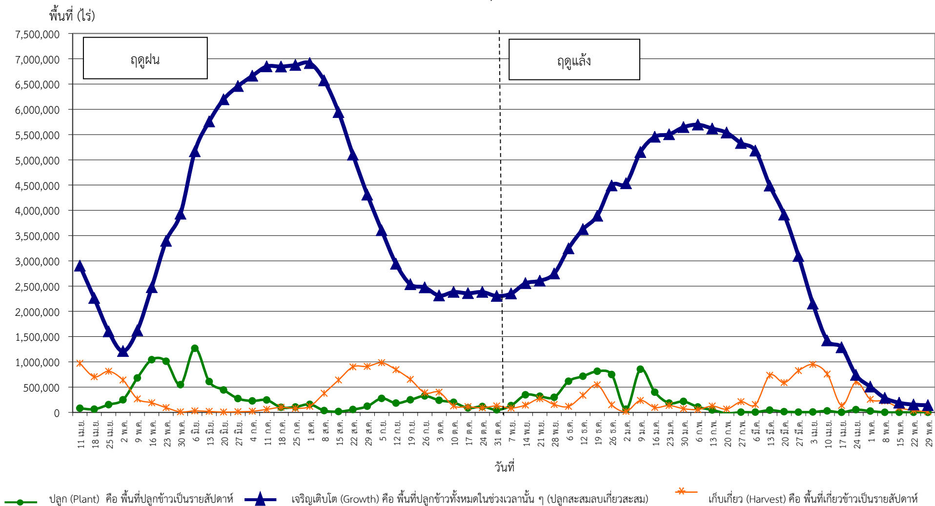
กราฟแสดงสภาพการปลูกข้าว ในเขตลุ่มน้ำเจ้าพระยาทำอย่างเก็บน้ำเขื่อนภูมิพลและสิริกิติ์ เป็นรายสัปดาห์ ณ วันที่ 29 พฤษภาคม 2562
