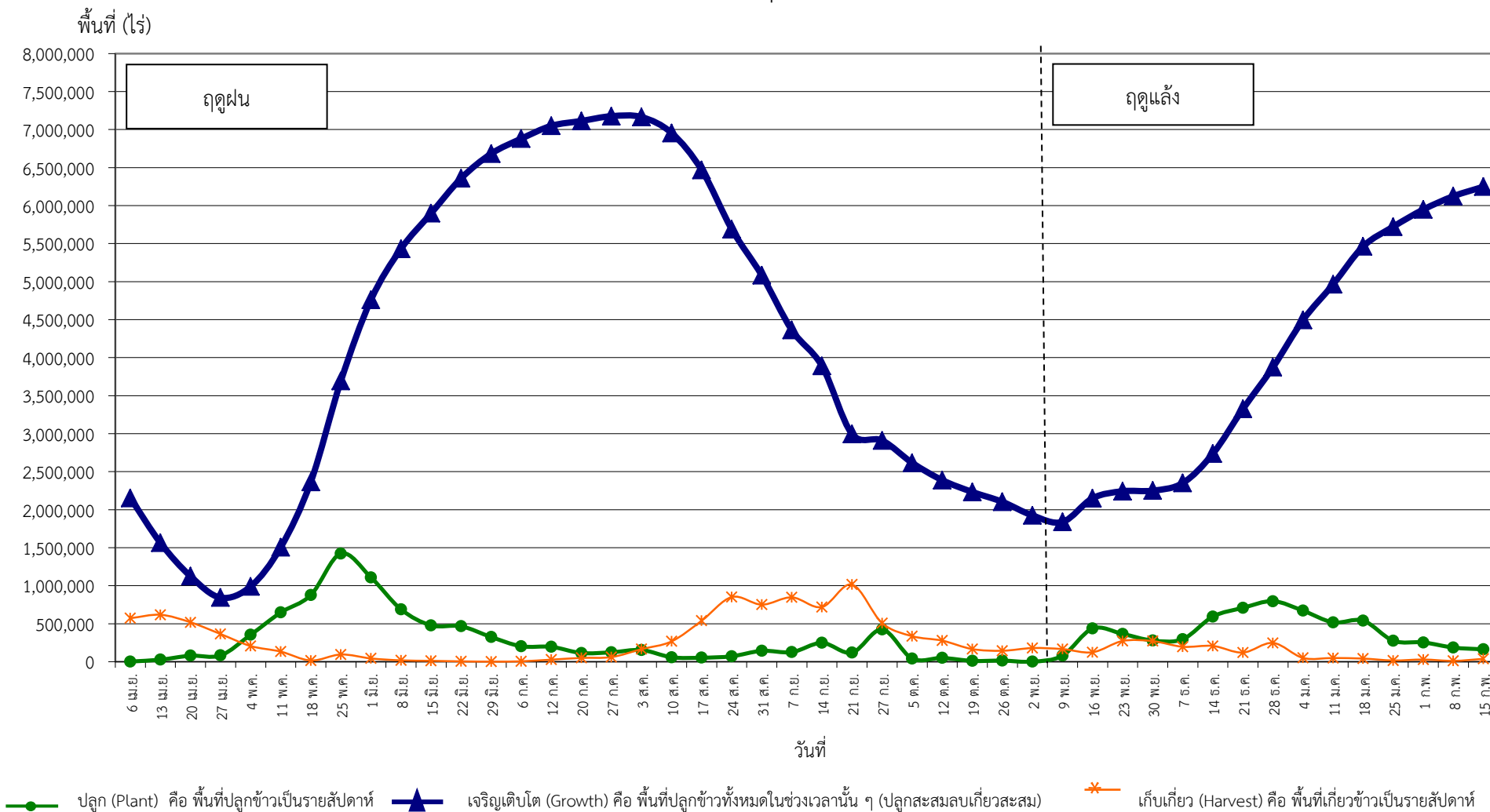
กราฟแสดงสภาพการปลูกข้าว ในเขตลุ่มน้ำเจ้าพระยาทำอย่างเก็บน้ำเขื่อนภูมิพลและสิริกิติ์ เป็นรายสัปดาห์ ณ วันที่ 15 กุมภาพันธ์ 2566
