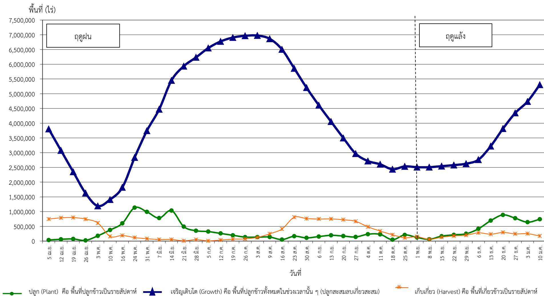
กราฟแสดงสภาพการปลูกข้าว ในเขตลุ่มน้ำเจ้าพระยาทำอย่างเก็บน้ำเขื่อนภูมิพลและสิริกิติ์ เป็นรายสัปดาห์ ณ วันที่ 10 มกราคม 2567
