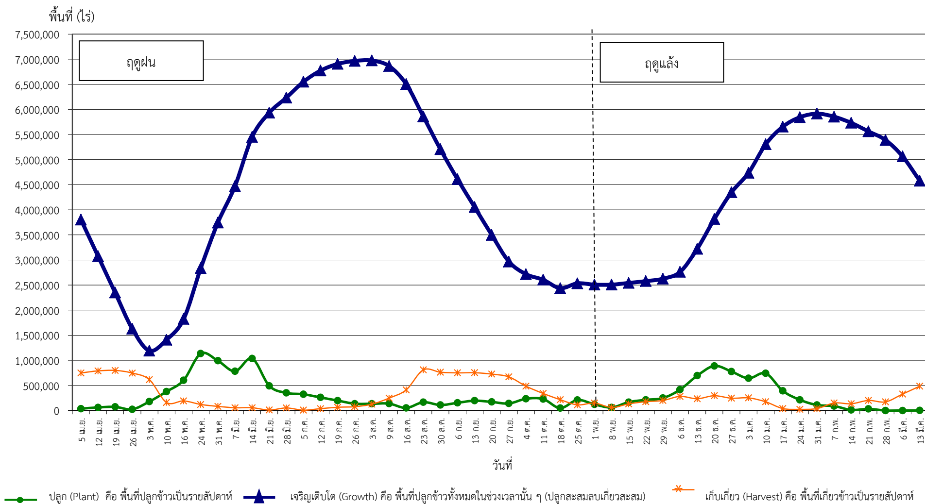
กราฟแสดงสภาพการปลูกข้าว ในเขตลุ่มน้ำเจ้าพระยาทำอย่างเก็บน้ำเขื่อนภูมิพลและสิริกิติ์ เป็นรายสัปดาห์ ณ วันที่ 13 มีนาคม 2567
