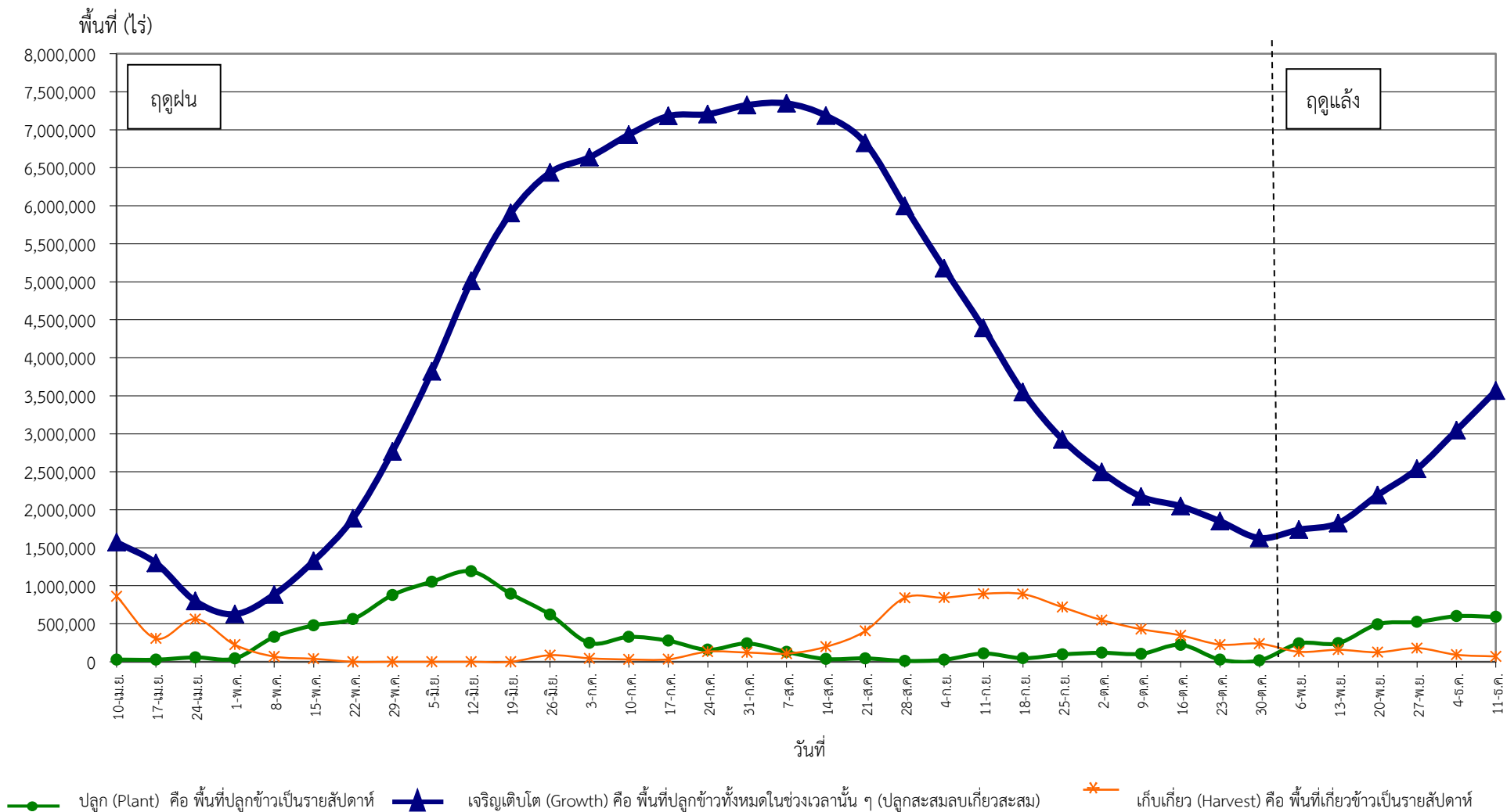
กราฟแสดงสภาพการปลูกข้าว ในเขตลุ่มน้ำเจ้าพระยาทำอย่างเก็บน้ำเขื่อนภูมิพลและสิริกิติ์ เป็นรายสัปดาห์ ณ วันที่ 11 ธันวาคม 2567
