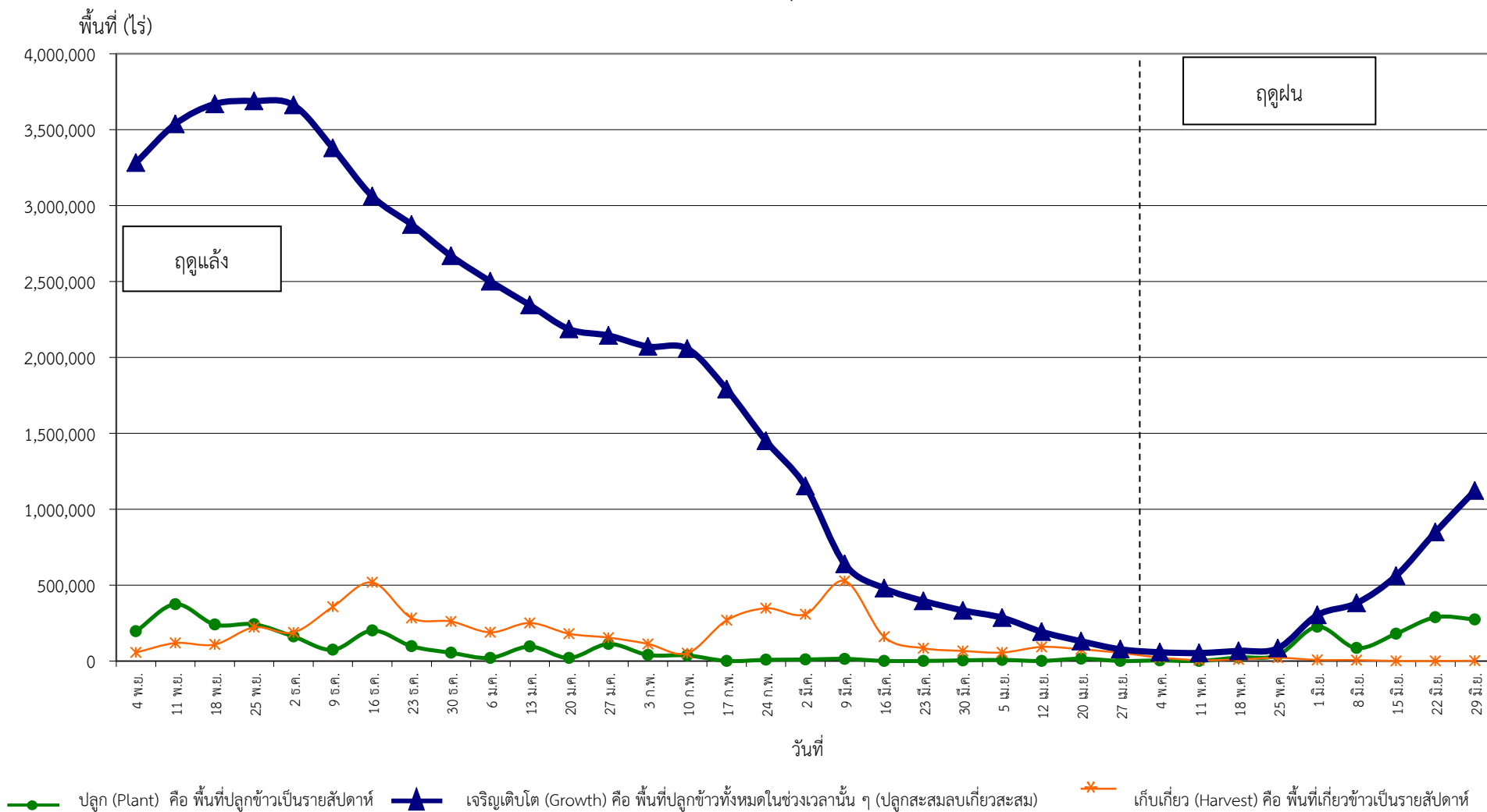
กราฟแสดงสภาพการปลูกข้าว ในเขตลุ่มน้ำเจ้าพระยาทำอย่างเก็บน้ำเขื่อนภูมิพลและสิริกิติ์ เป็นรายสัปดาห์ ณ วันที่ 29 มิถุนายน 2559
