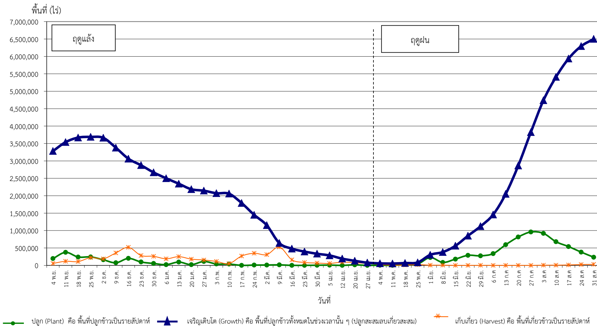
กราฟแสดงสภาพการปลูกข้าว ในเขตลุ่มน้ำเจ้าพระยาทำอย่างเก็บน้ำเขื่อนภูมิพลและสิริกิติ์ เป็นรายสัปดาห์ ณ วันที่ 31 สิงหาคม 2559
