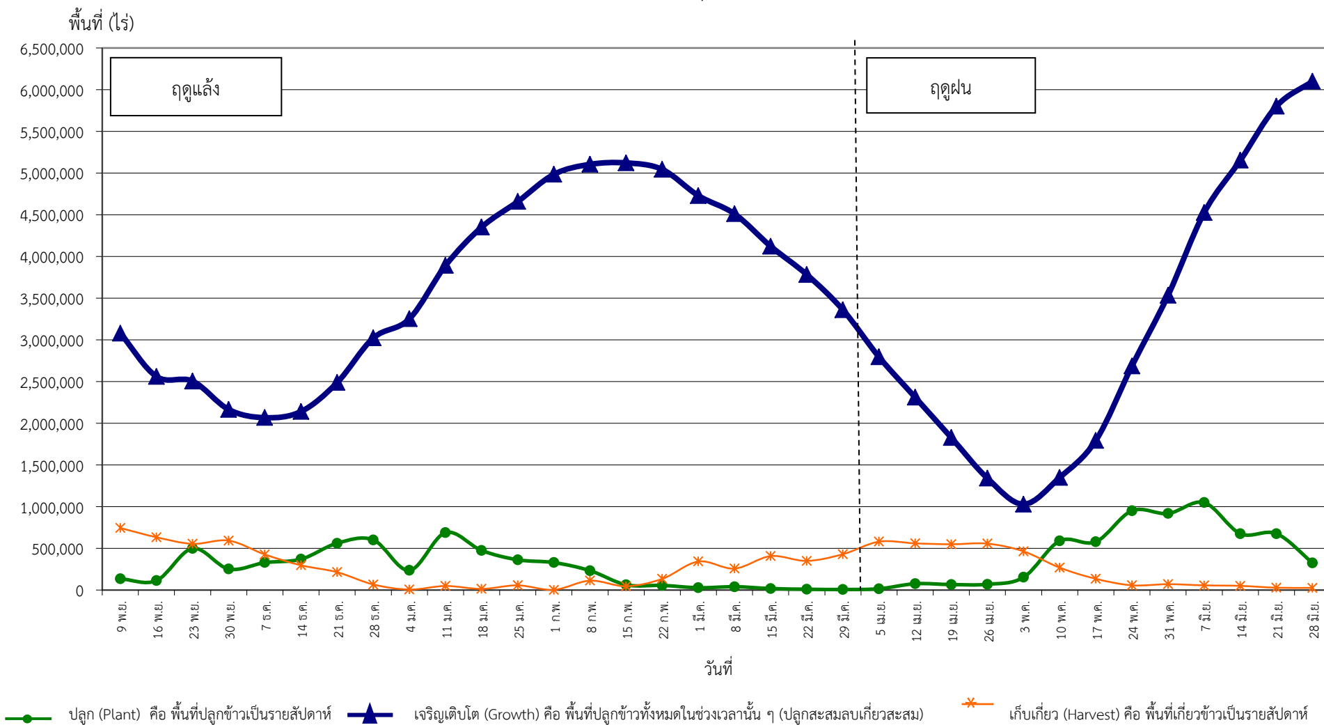
กราฟแสดงสภาพการปลูกข้าว ในเขตลุ่มน้ำเจ้าพระยาทำอย่างเก็บน้ำเขื่อนภูมิพลและสิริกิติ์ เป็นรายสัปดาห์ ณ วันที่ 28 มิถุนายน 2560
