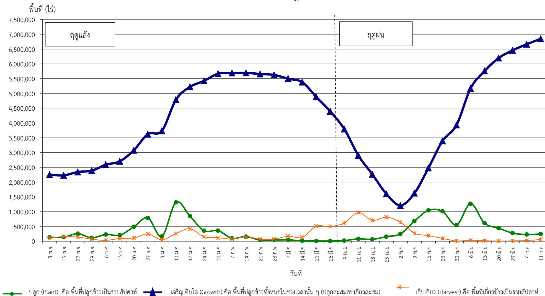
กราฟแสดงสภาพการปลูกข้าว ในเขตลุ่มน้ำเจ้าพระยาทำอย่างเก็บน้ำเขื่อนภูมิพลและสิริกิติ์ เป็นรายสัปดาห์ ณ วันที่ 11 กรกฎาคม 2561
