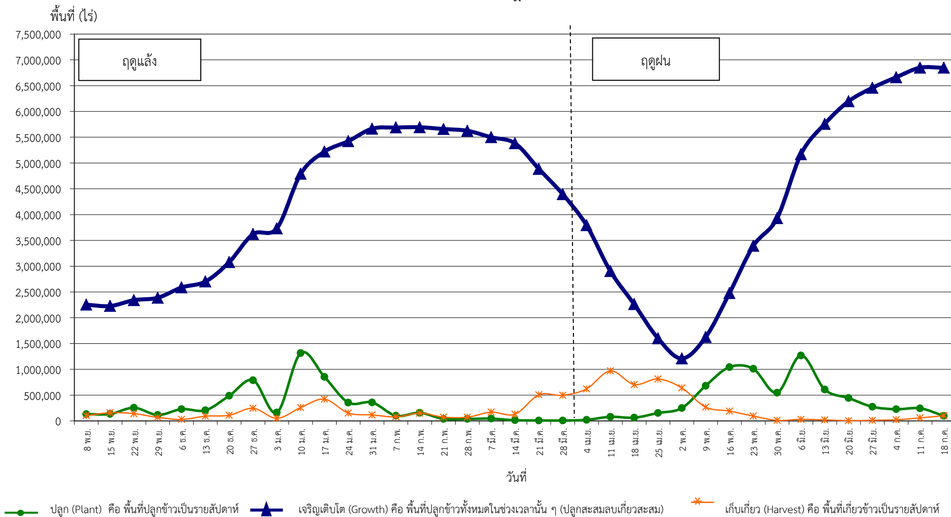
กราฟแสดงสภาพการปลูกข้าว ในเขตลุ่มน้ำเจ้าพระยาทำอย่างเก็บน้ำเขื่อนภูมิพลและสิริกิติ์ เป็นรายสัปดาห์ ณ วันที่ 18 กรกฎาคม 2561
