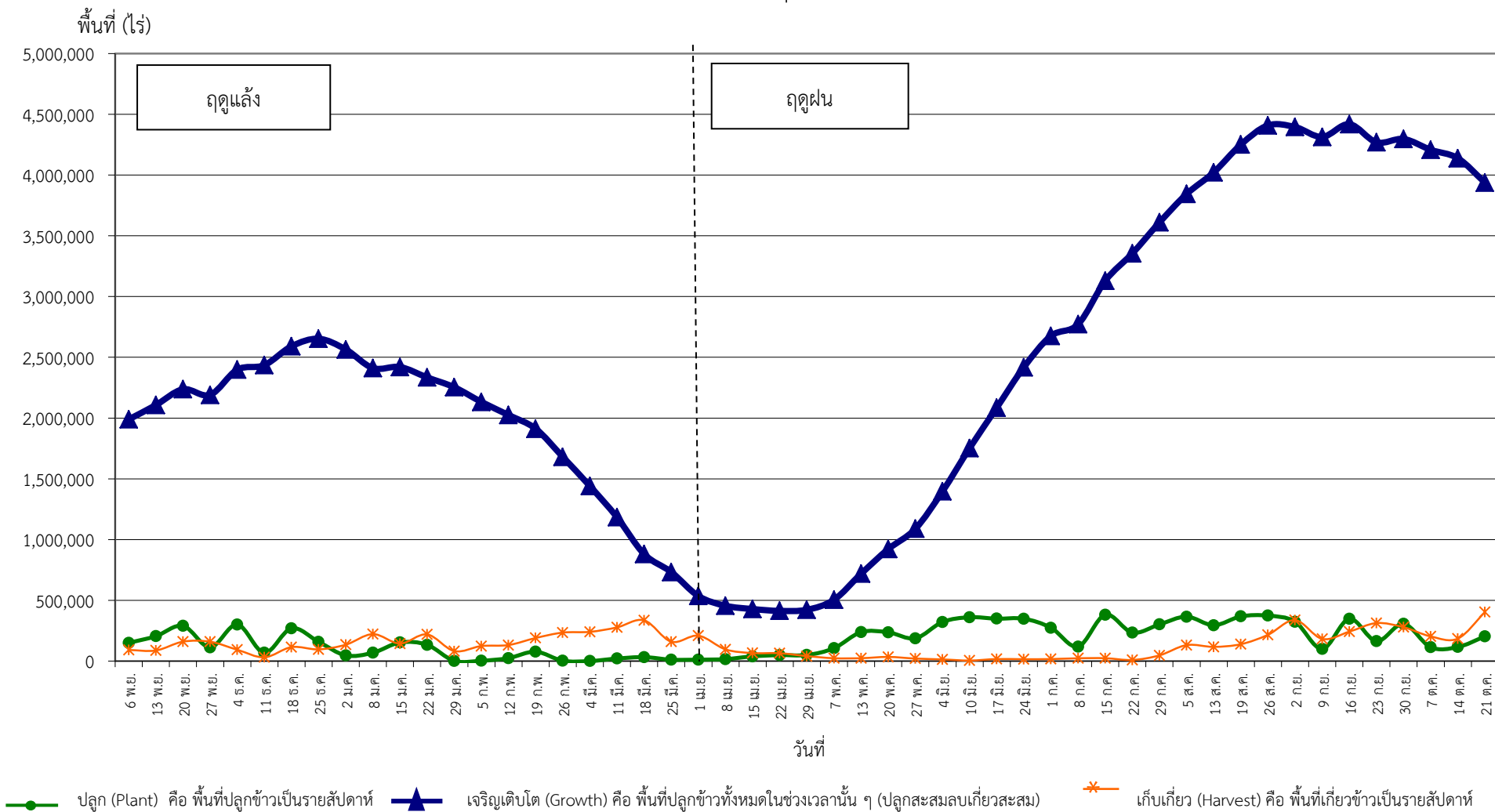
กราฟแสดงสภาพการปลูกข้าว ในเขตลุ่มน้ำเจ้าพระยาทำอย่างเก็บน้ำเขื่อนภูมิพลและสิริกิติ์ เป็นรายสัปดาห์ ณ วันที่ 21 ตุลาคม 2563
