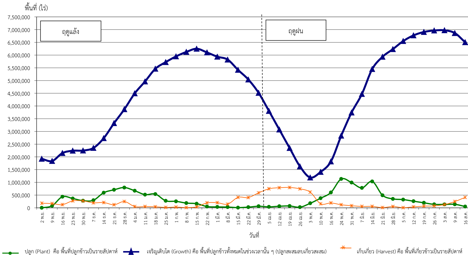
กราฟแสดงสภาพการปลูกข้าว ในเขตลุ่มน้ำเจ้าพระยาทำอย่างเก็บน้ำเขื่อนภูมิพลและสิริกิติ์ เป็นรายสัปดาห์ ณ วันที่ 16 สิงหาคม 2566
