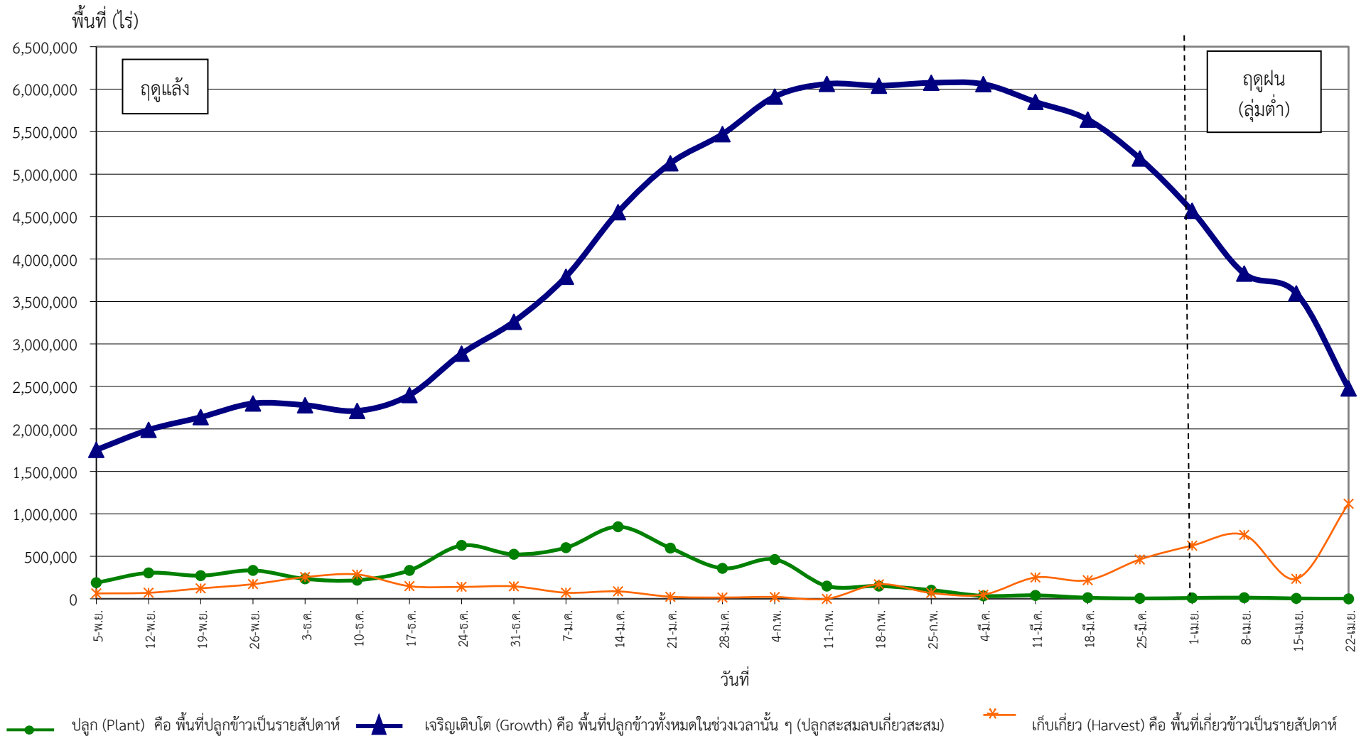
กราฟแสดงสภาพการปลูกข้าว ในเขตลุ่มน้ำเจ้าพระยาทำอย่างเก็บน้ำเขื่อนภูมิพลและสิริกิติ์ เป็นรายสัปดาห์ ณ วันที่ 22 เมษายน 2568
