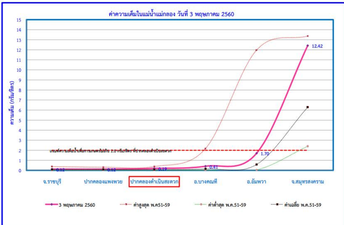
รูปที่ 16 ค่าความเค็มในแม่น้ำแม่กลอง วันที่3 พฤษภาคม พ.ศ. 2560
