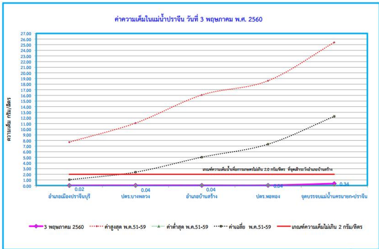
รูปที่ 23 ค่าความเค็มในแม่น้ำปราจีนบุรี วันที่ 3 พฤษภาคม พ.ศ. 2560
