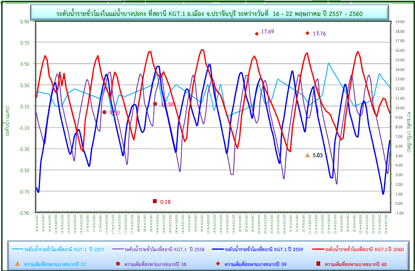
รูปที่ 21 ระดับน้ำรายชั่วโมงที่สถานี KGT.1 และความเค็มที่สะพานบางซอก
