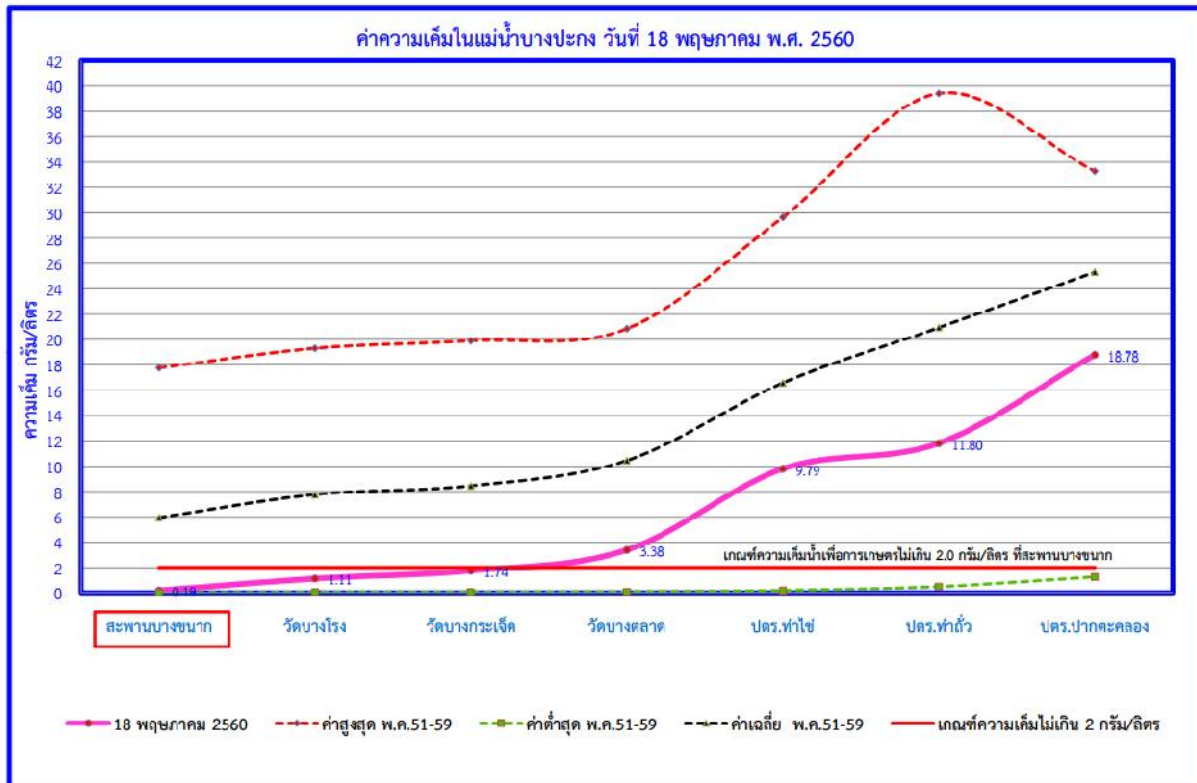
รูปที่ 20 ค่าความเค็มในแม่น้ำบางปะกง วันที่ 18 พฤษภาคม พ.ศ. 2560
