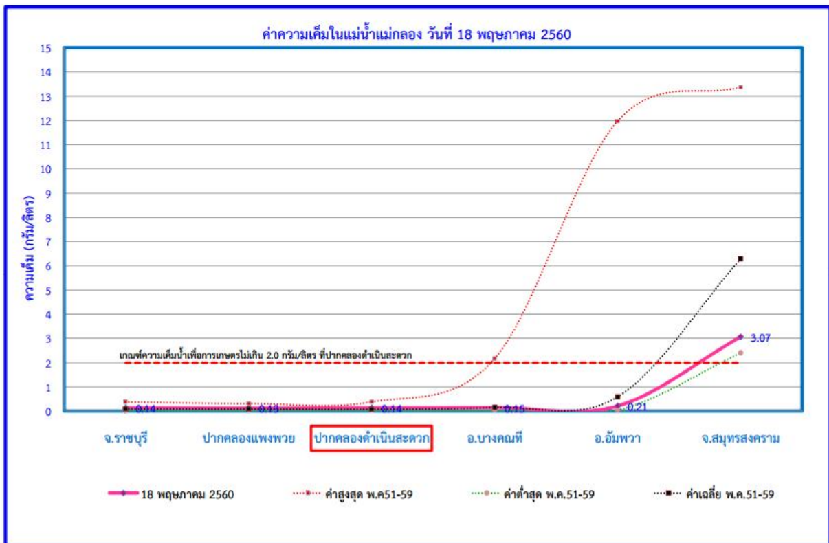
รูปที่ 16 ค่าความเค็มในแม่น้ำแม่กลอง วันที่ 18 พฤษภาคม พ.ศ. 2560
