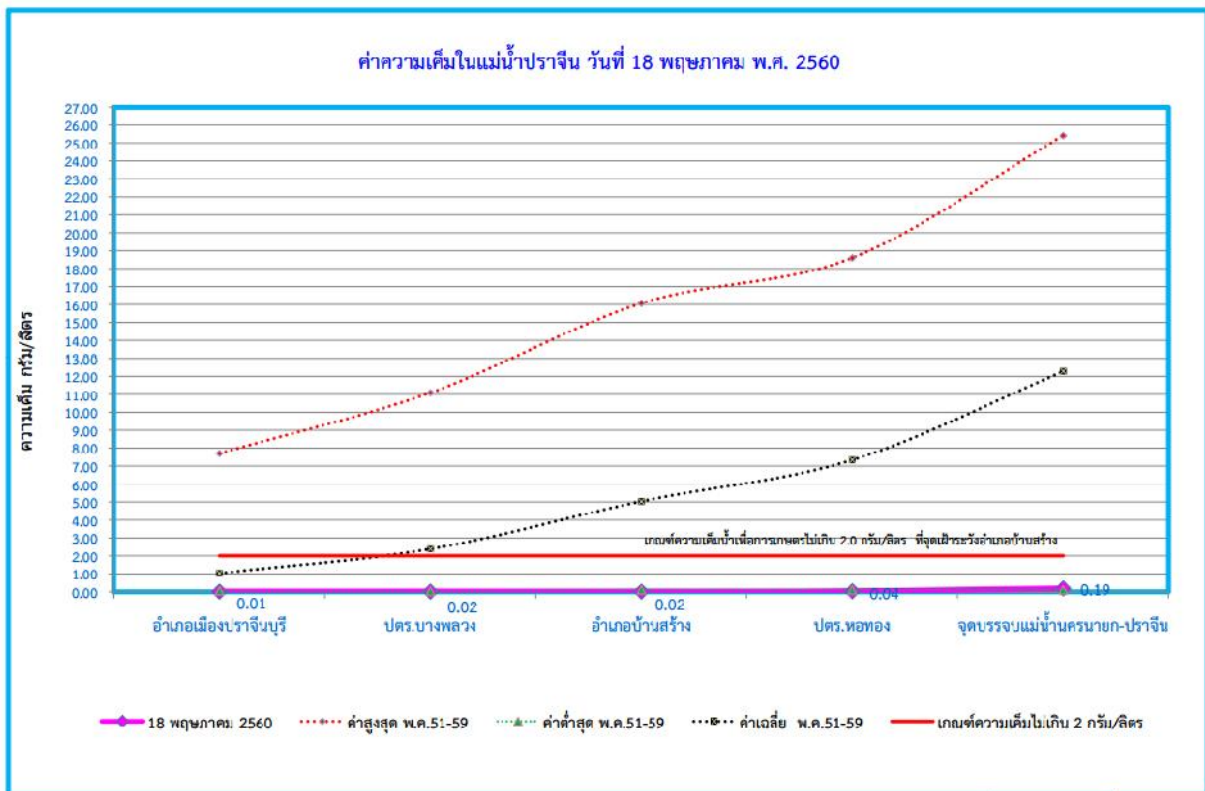
รูปที่ 23 ค่าความเค็มในแม่น้ำปราจีนบุรี วันที่ 18 พฤษภาคม พ.ศ. 2560
