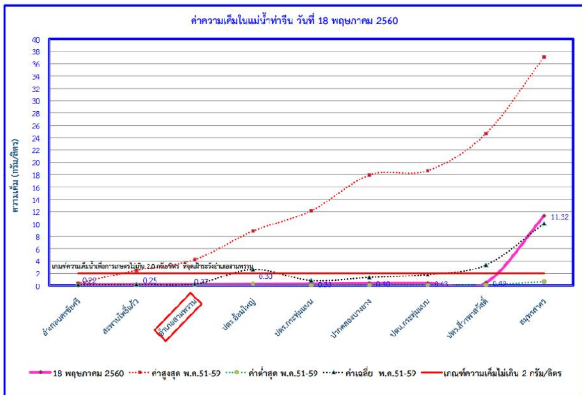
รูปที่ 12 ค่าความเค็มในแม่น้ำท่าจีน วันที่ 18 พฤษภาคม พ.ศ. 2560
