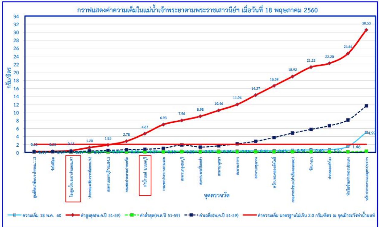
รูปที่ 4 ค่าความเค็มในแม่น้ำเจ้าพระยา วันที่ 18 พฤษภาคม พ.ศ. 2560
