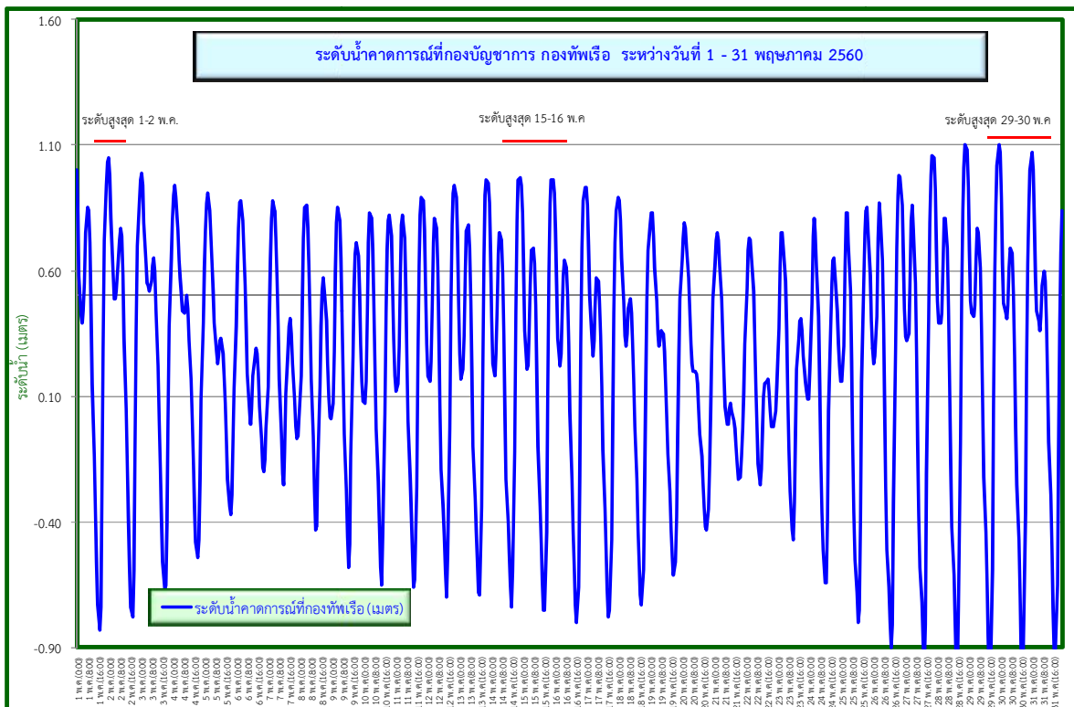
รูปที่ 11 ระดับน้ำคาดการณ์ที่กองบัญชาการกองทัพเรือโดยกรมอุทกศาสตร์ กองทัพเรือ
