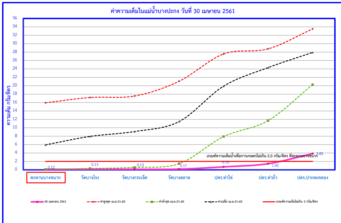
รูปที่ 18 ค่าความเค็มในแม่น้ำบางปะกง วันที่ 30 เมษายน พ.ศ. 2561
