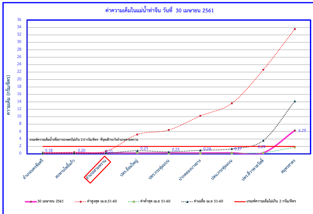
รูปที่ 10 ค่าความเค็มในแม่น้ำท่าจีน วันที่ 30 เมษายน พ.ศ. 2561
