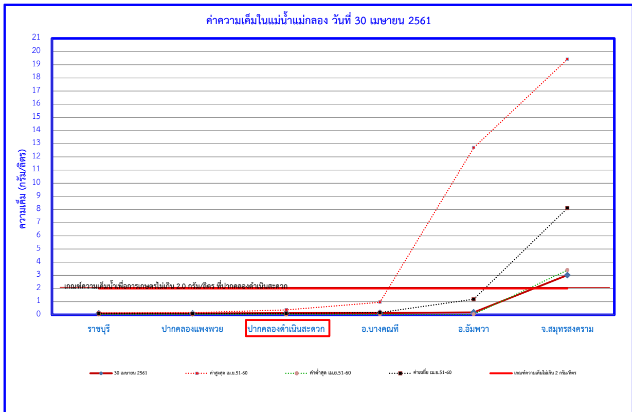
รูปที่ 14 ค่าความเค็มในแม่น้ำแม่กลอง วันที่ 30 เมษายน พ.ศ. 2561
