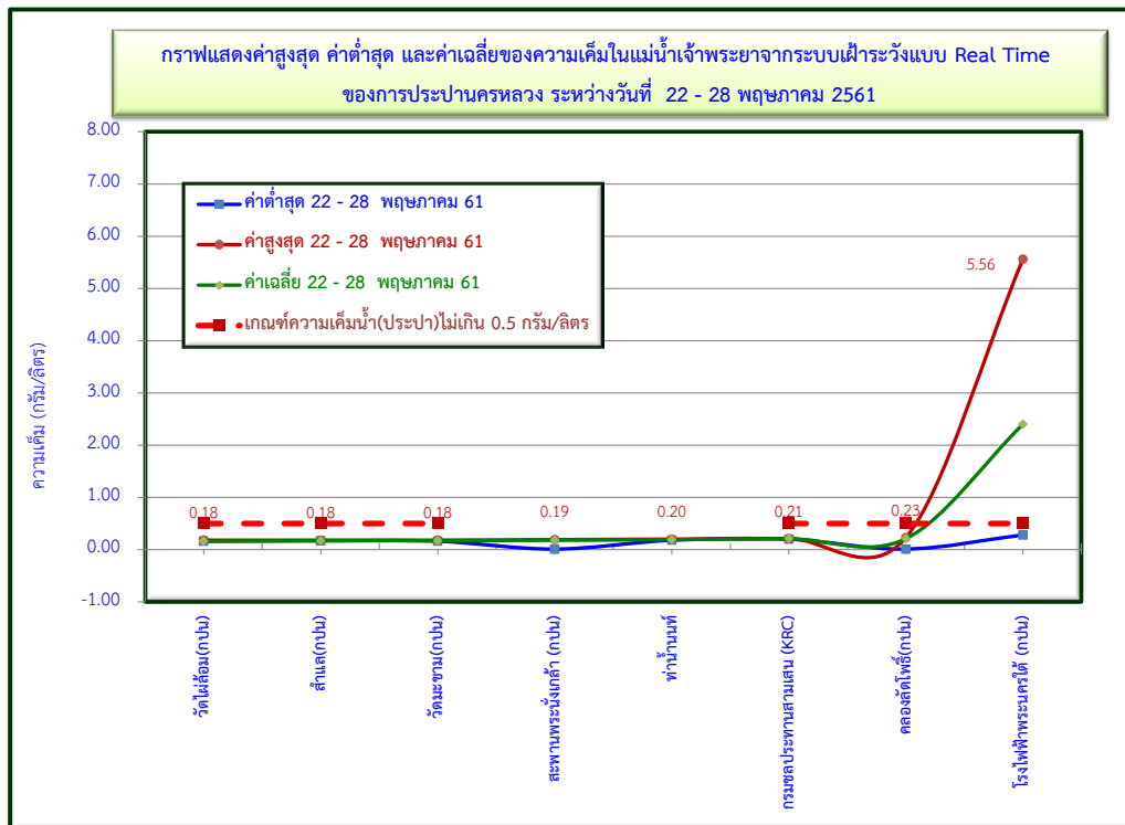
รูปที่ 4 กราฟแสดงความเค็มในแม่น้ำเจ้าพระยาจากระบบเฝ้าระวังแบบ Real Time
