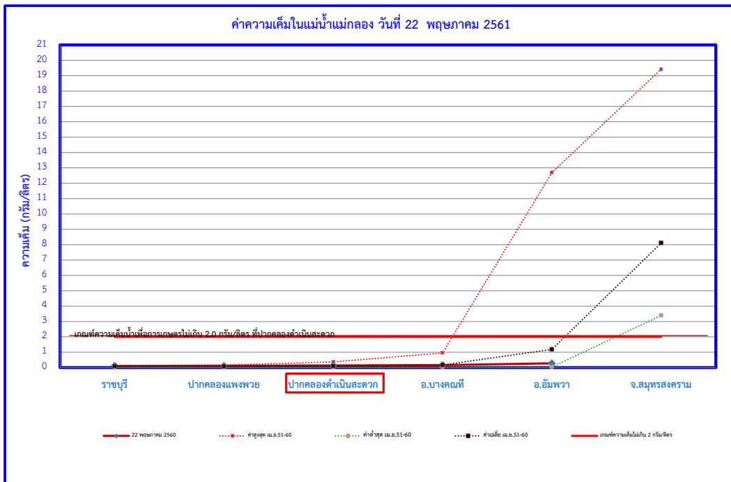
รูปที่ 14 ค่าความเค็มในแม่น้ำแม่กลอง วันที่ 22 พฤษภาคม พ.ศ. 2561
