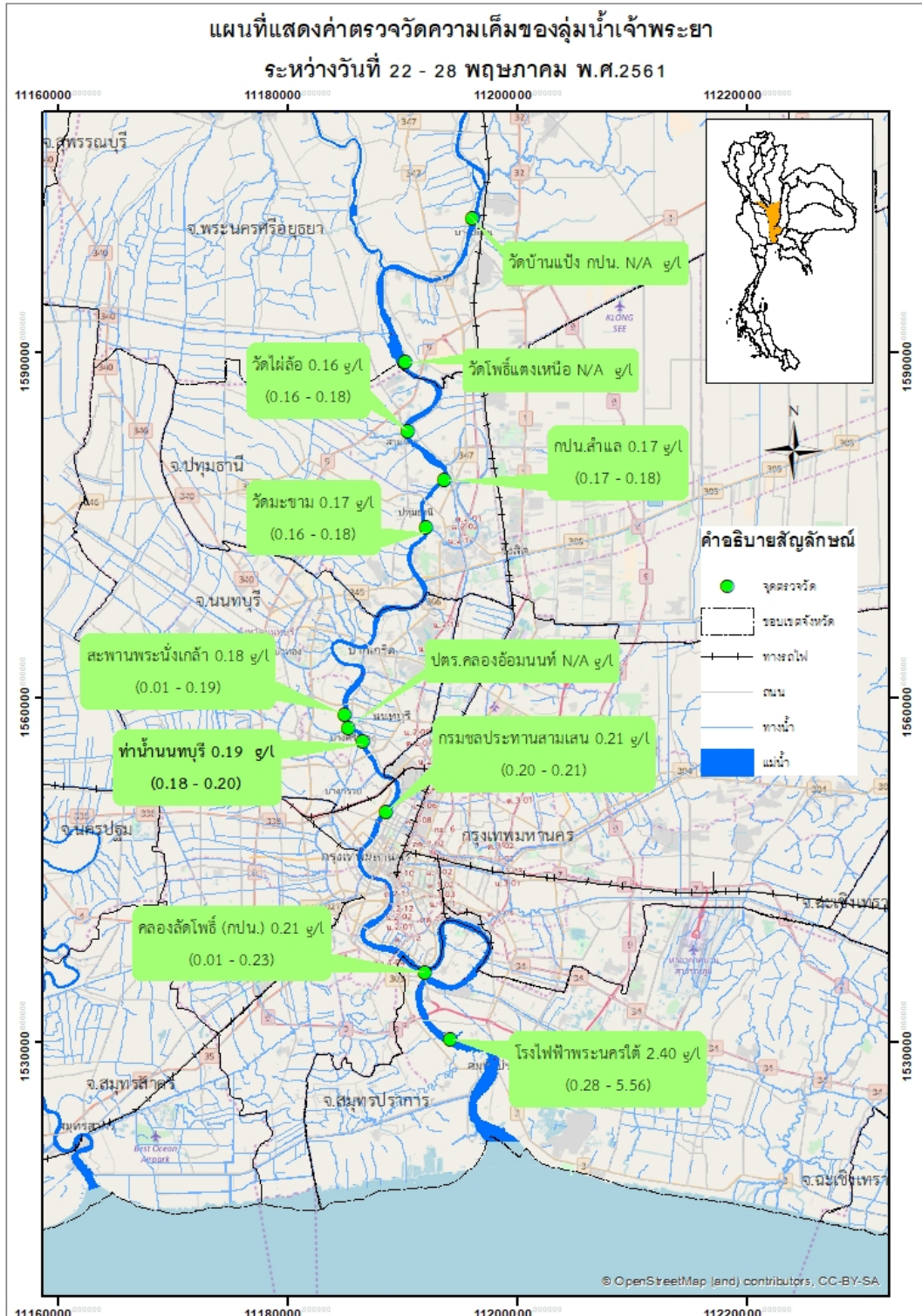
รูปที่ 5 ความเค็มในแม่น้ำเจ้าพระยา
