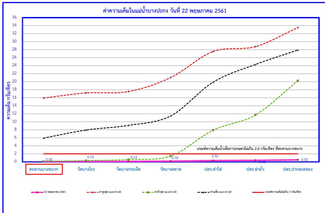
รูปที่ 18 ค่าความเค็มในแม่น้ำบางปะกง วันที่ 22 พฤษภาคม พ.ศ. 2561
