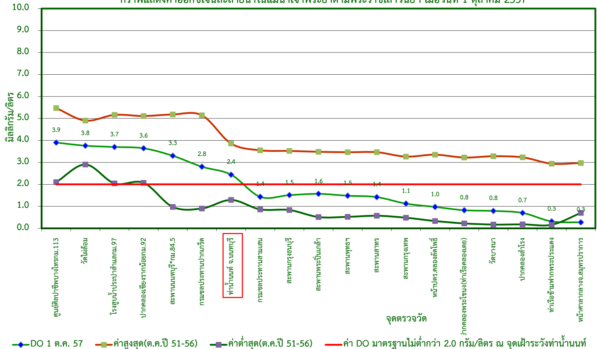
กราฟแสดงค่าออกซิเจนละลายน้ำในแม่น้ำเจ้าพระยาตามพระราชเสาวนีย์ฯ เมื่อวันที่ 1 ตุลาคม 2557
