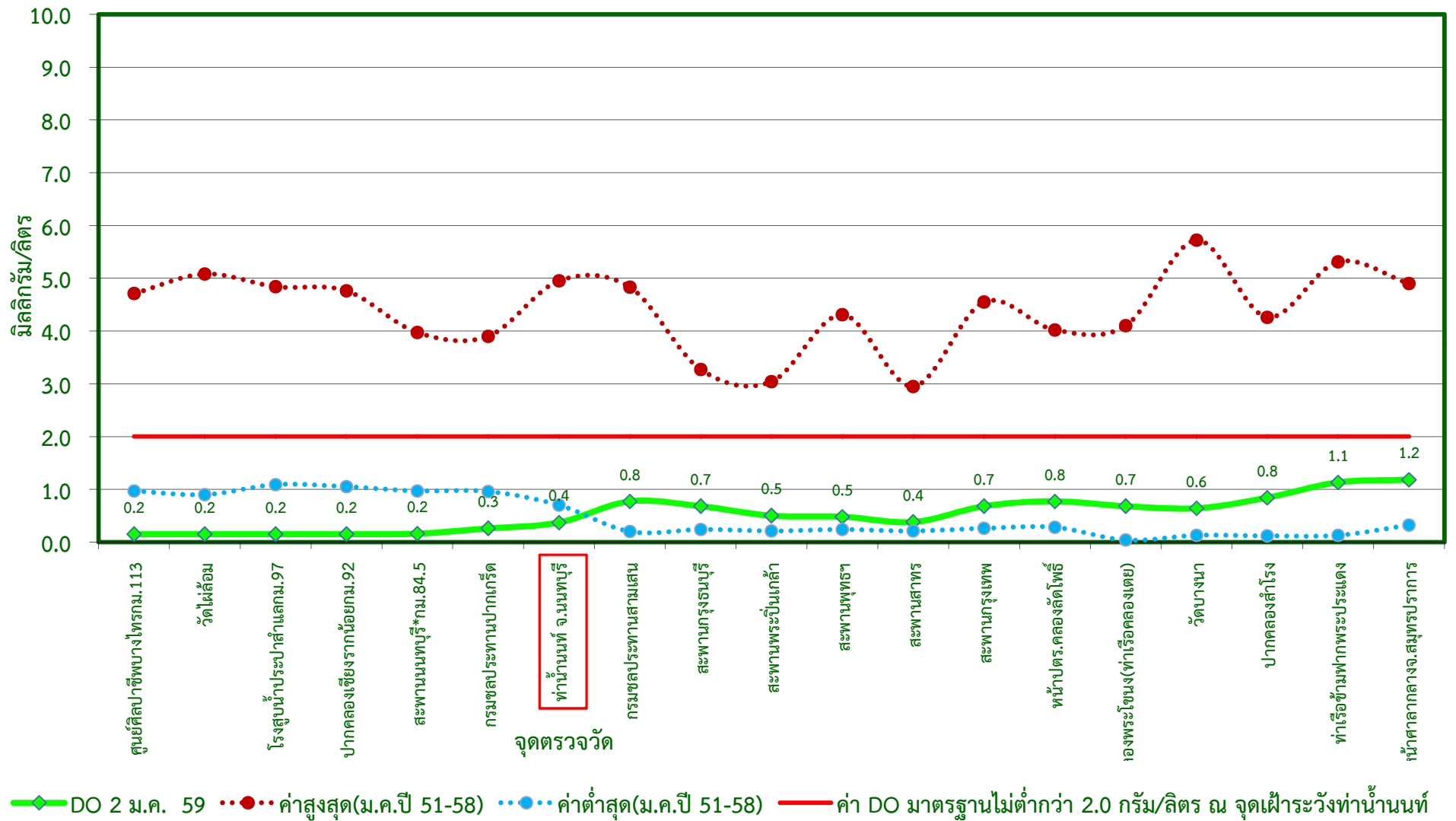
กราฟแสดงค่าออกซิเจนละลายน้ำในแม่น้ำเจ้าพระยาตามพระราชเสาวนีย์ฯ เมื่อวันที่ 2 มกราคม 2559
