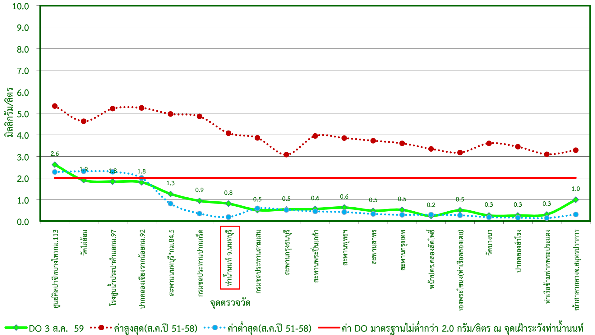
กราฟแสดงค่าออกซิเจนละลายน้ำในแม่น้ำเจ้าพระยาตามพระราชเสาวนีย์ฯ เมื่อวันที่ 3 สิงหาคม 2559
