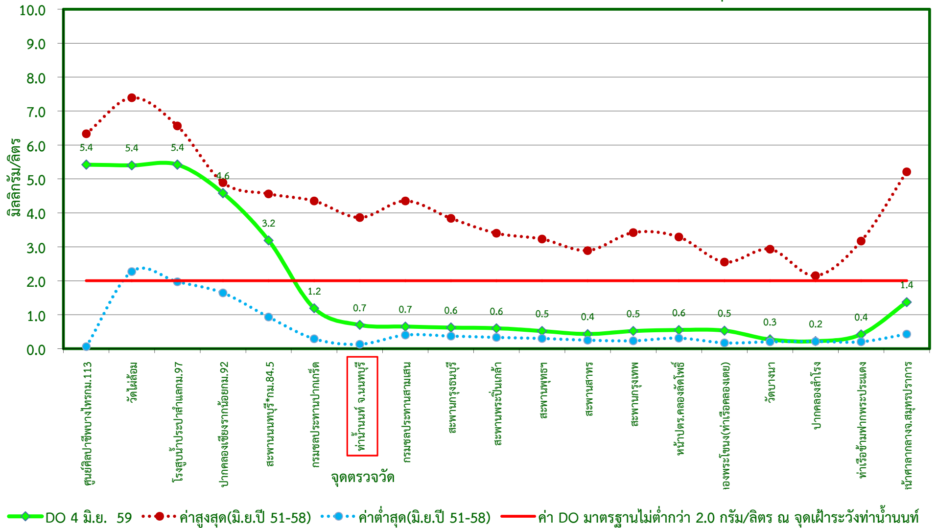
กราฟแสดงค่าออกซิเจนละลายน้ำในแม่น้ำเจ้าพระยาตามพระราชเสาวนีย์ฯ เมื่อวันที่ 4 มิถุนายน 2559
