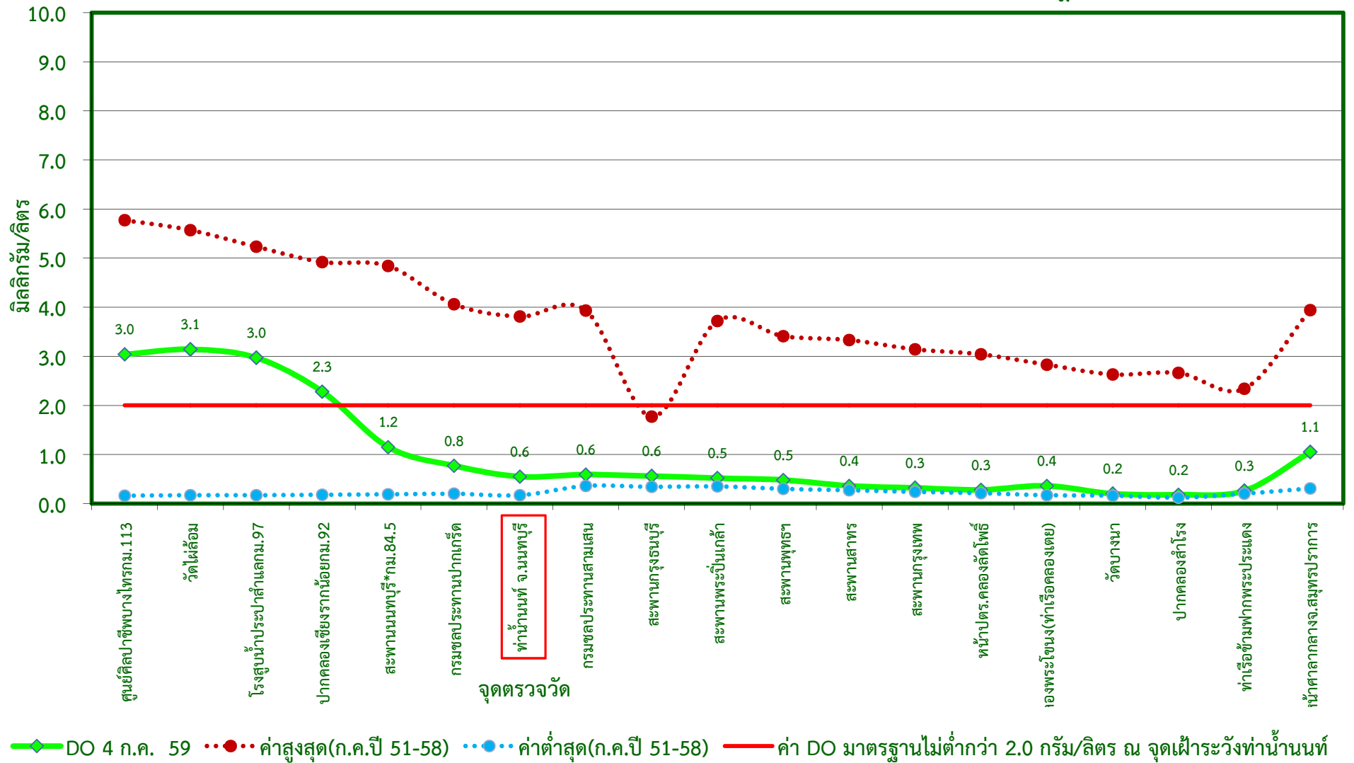
กราฟแสดงค่าออกซิเจนละลายน้ำในแม่น้ำเจ้าพระยาตามพระราชเสาวนีย์ฯ เมื่อวันที่ 4 กรกฎาคม 2559
