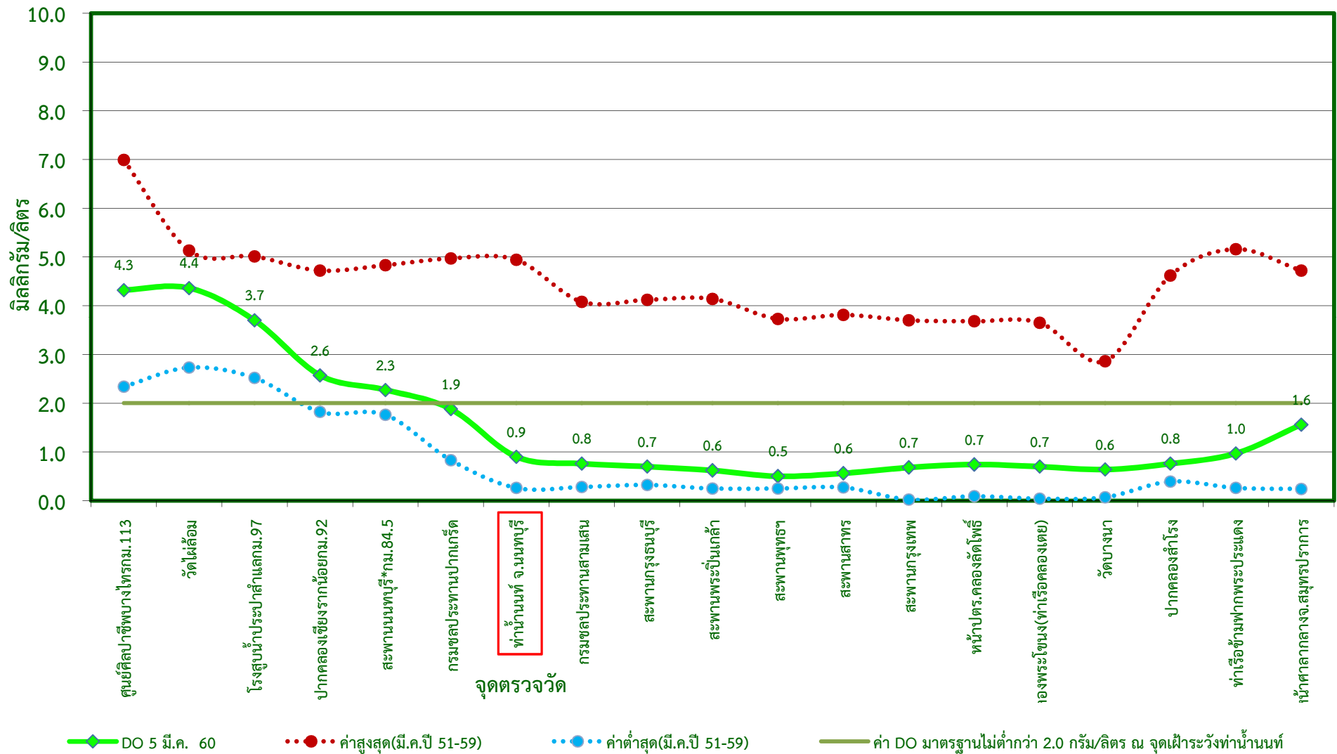
กราฟแสดงค่าออกซิเจนละลายน้ำในแม่น้ำเจ้าพระยาตามพระราชเสาวนีย์ฯ เมื่อวันที่ 5 มีนาคม 2560
