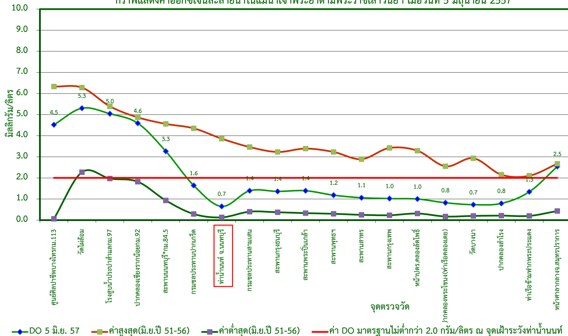
กราฟแสดงค่าออกซิเจนละลายน้ำในแม่น้ำเจ้าพระยาตามพระราชเสาวนีย์ฯ เมื่อวันที่ 5 มิถุนายน 2557
