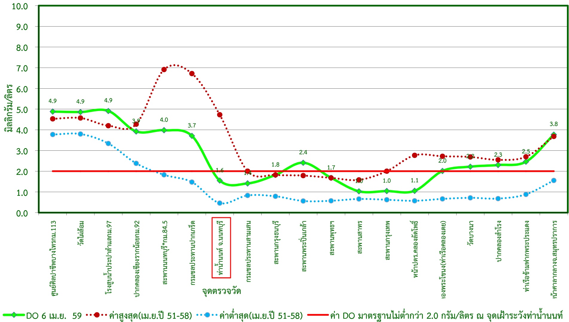
กราฟแสดงค่าออกซิเจนละลายน้ำในแม่น้ำเจ้าพระยาตามพระราชเสาวนีย์ฯ เมื่อวันที่ 6 เมษายน 2559
