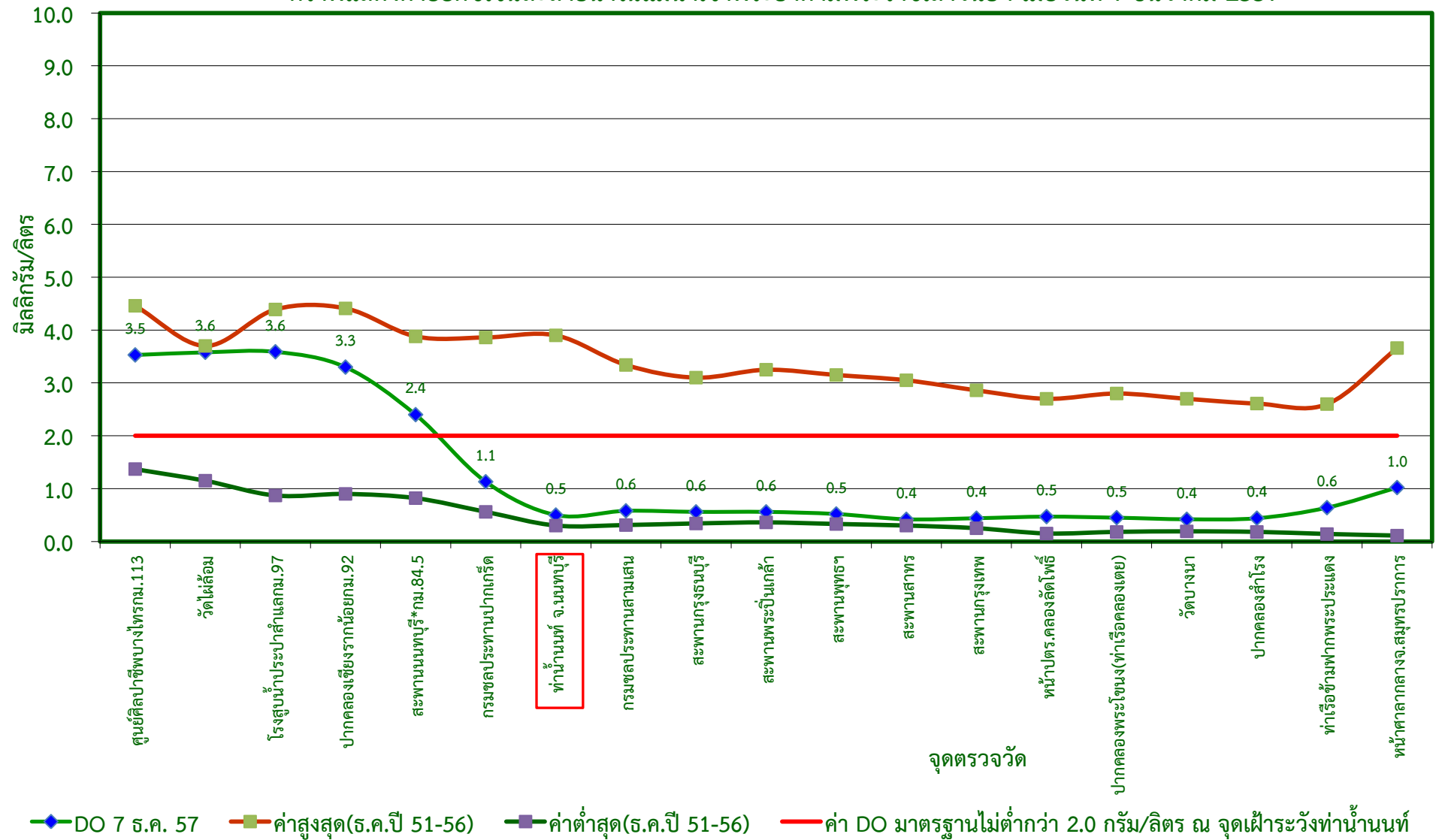
กราฟแสดงค่าออกซิเจนละลายน้ำในแม่น้ำเจ้าพระยาตามพระราชเสาวนีย์ฯ เมื่อวันที่ 7 ธันวาคม 2557
