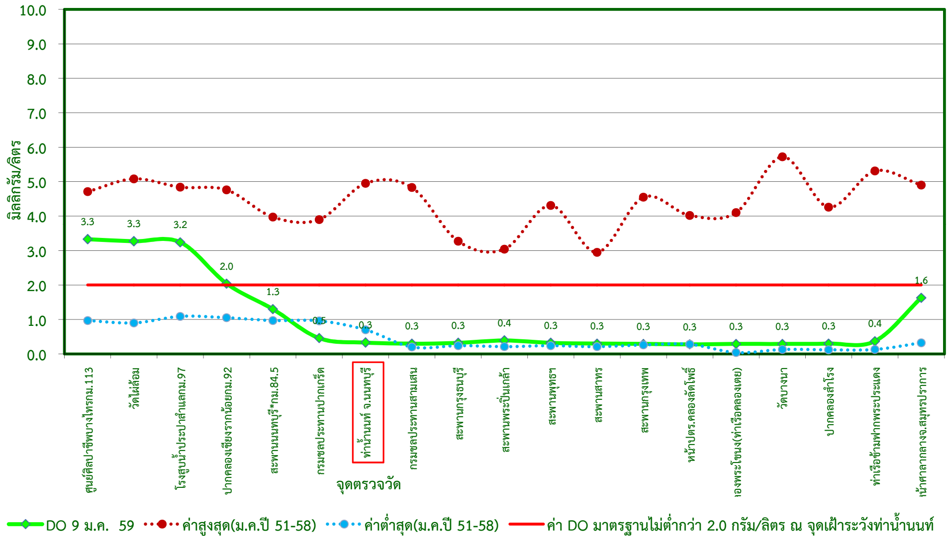
กราฟแสดงค่าออกซิเจนละลายน้ำในแม่น้ำเจ้าพระยาตามพระราชเสาวนีย์ฯ เมื่อวันที่ 9 มกราคม 2559
