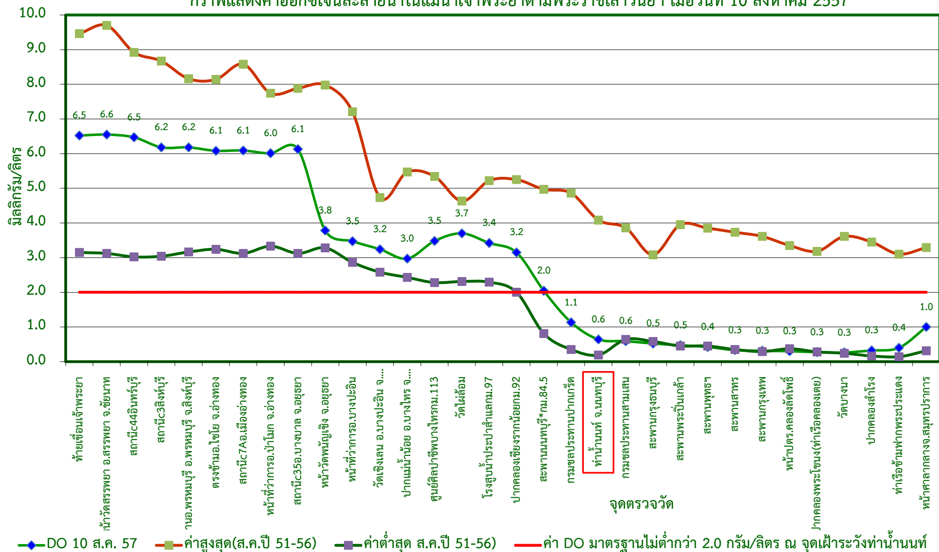
กราฟแสดงค่าออกซิเจนละลายน้ำในแม่น้ำเจ้าพระยาตามพระราชเสาวนีย์ฯ เมื่อวันที่ 10 สิงหาคม 2557
