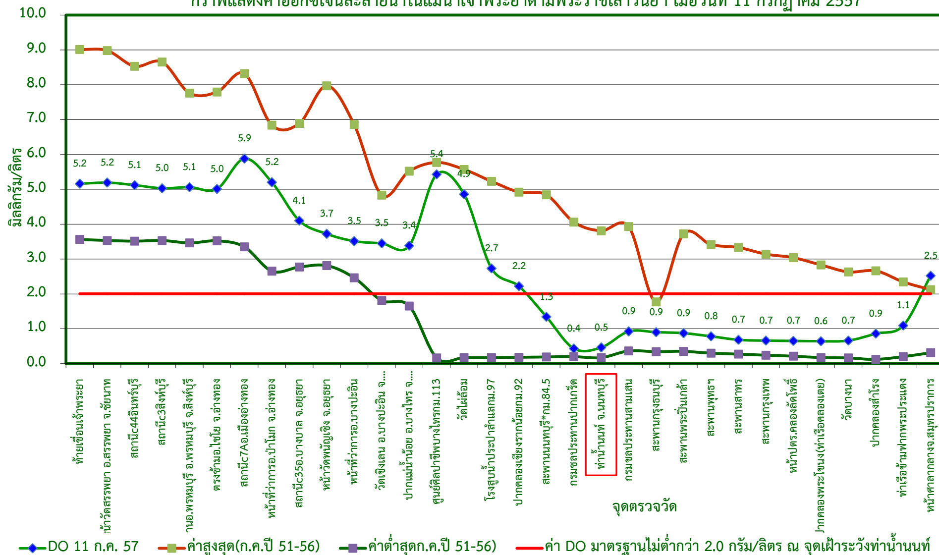
กราฟแสดงค่าออกซิเจนละลายน้ำในแม่น้ำเจ้าพระยาตามพระราชเสาวนีย์ฯ เมื่อวันที่ 11 กรกฎาคม 2557
