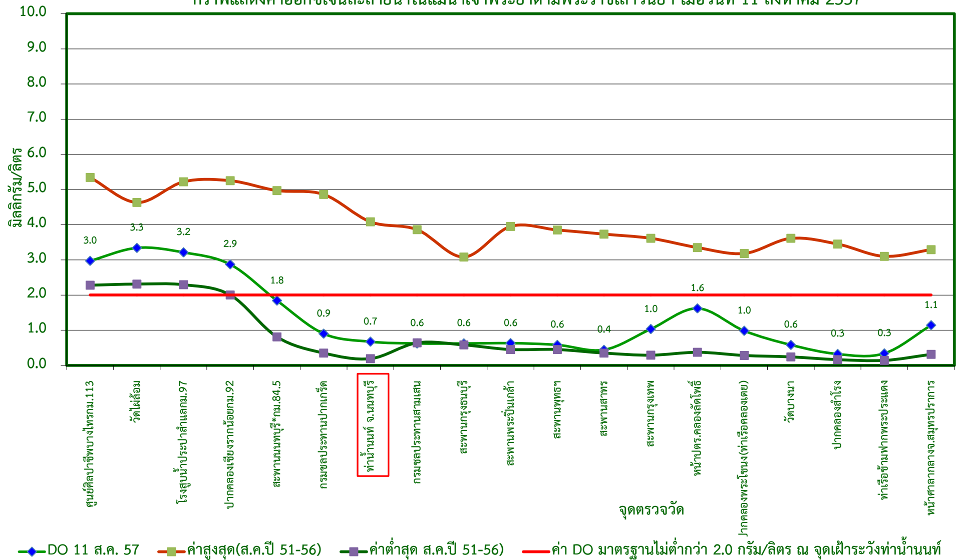
กราฟแสดงค่าออกซิเจนละลายน้ำในแม่น้ำเจ้าพระยาตามพระราชเสาวนีย์ฯ เมื่อวันที่ 11 สิงหาคม 2557
